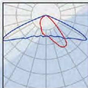
Диаграмма КСС типа Ш (широкая)
