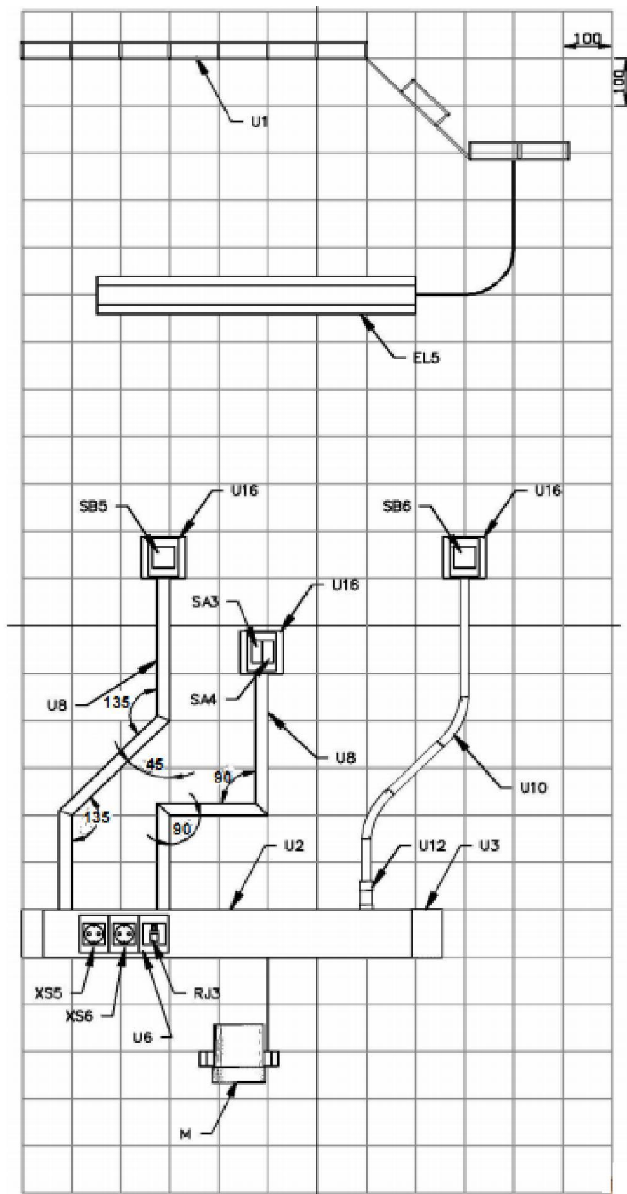
Монтажная схема. Вид «В»
