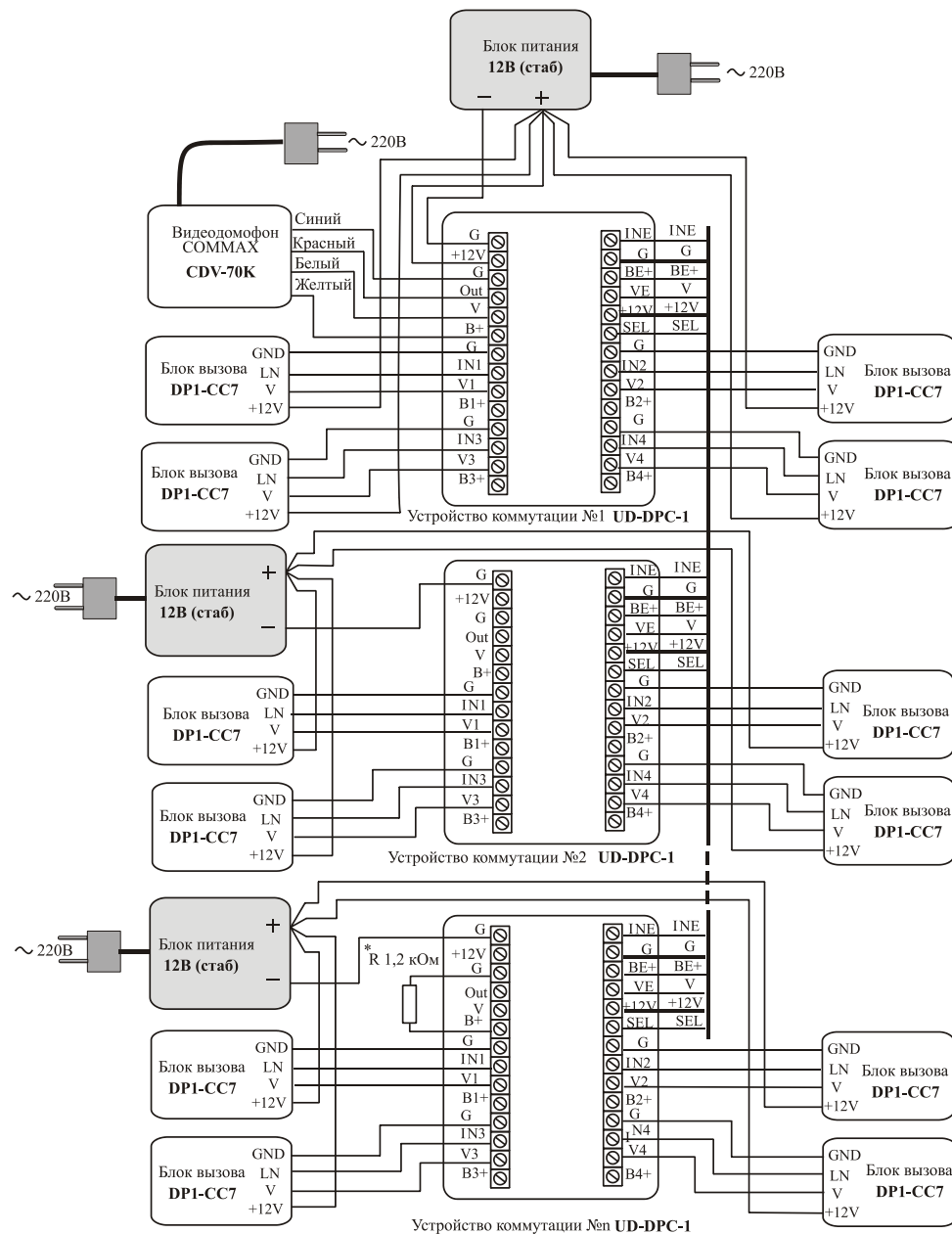
Рис.2 Схема соединения устройств коммутации
