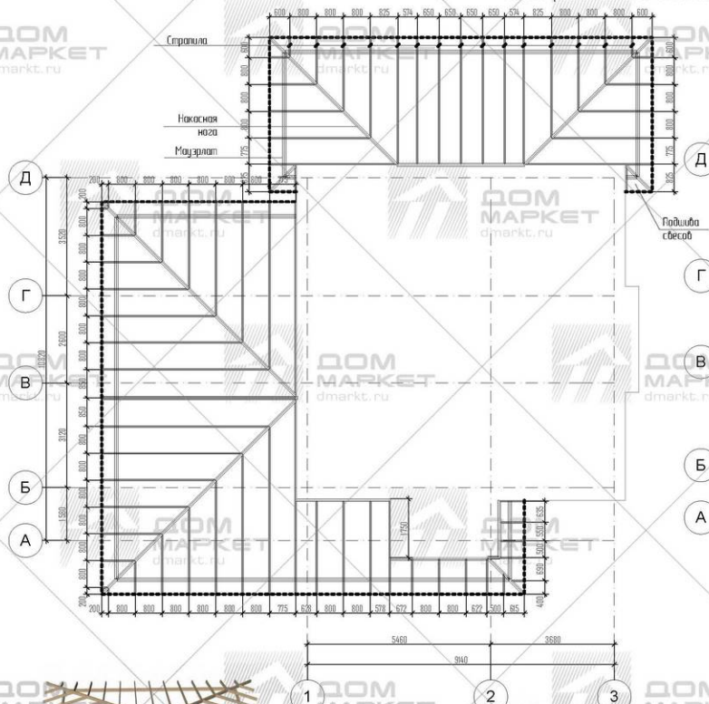
Схема расположения элементов стропильной системы
