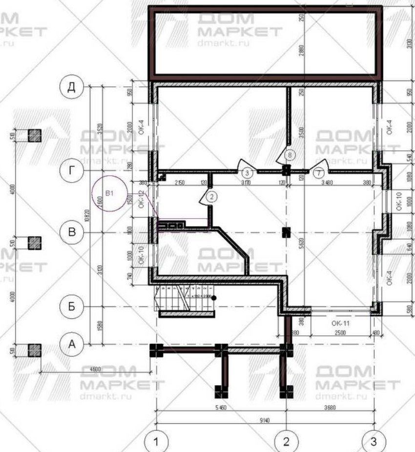
План отделки цоколя
