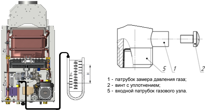
Рис. 7. Подключение дифманометра
