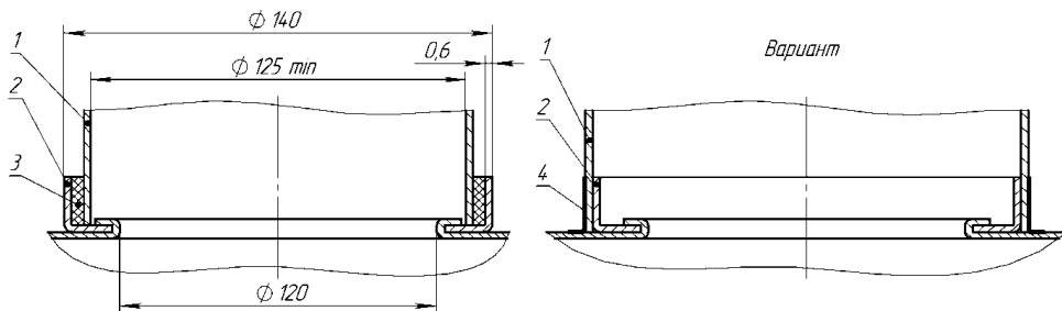
Рис. 4. Схема подсоединения газоотводящей трубы
