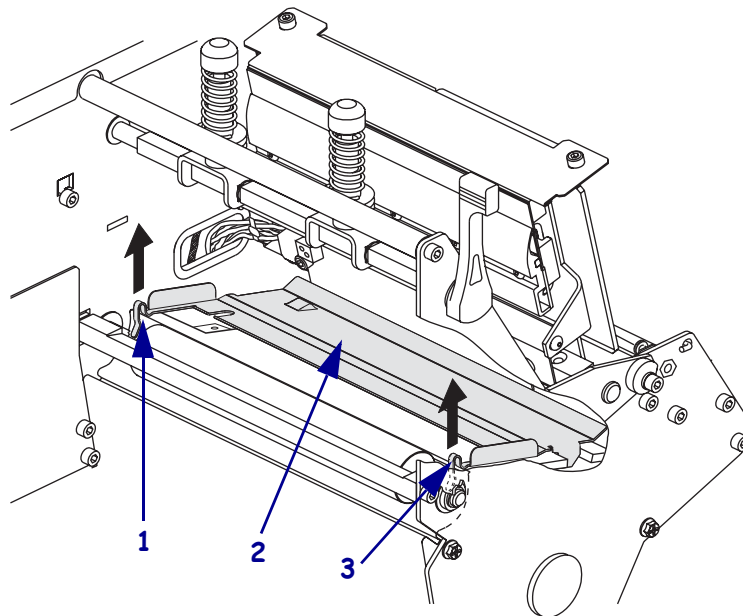
Рис. 20 • Расположение держателя
