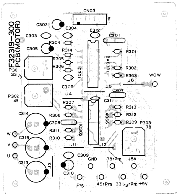
55-1 Motor PCB
