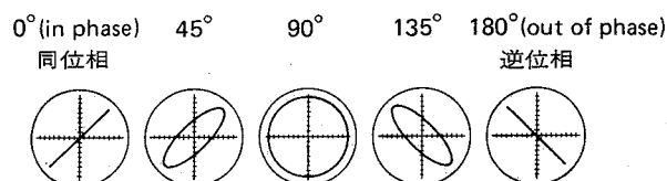
Fig. 4-5 Confirming phase relationship 位相関係図
