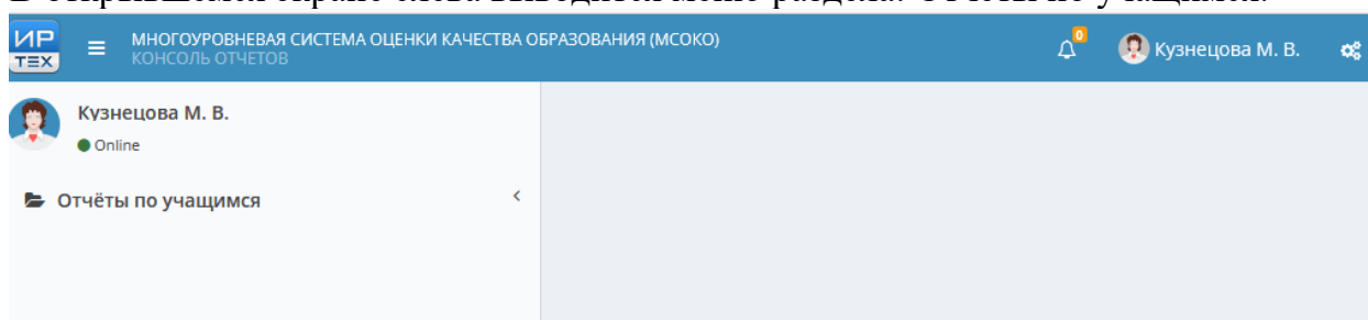
Рисунок 2 – Модуль МСОКО
