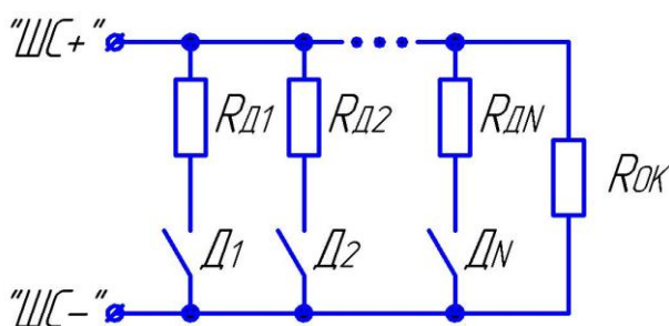
Рис.4 Схема подключения проводных пожарных дымовых датчиков к шлейфу с типом =7 (Д1...ДN – контакты пожарных дымовых датчиков; Rок – оконечный резистор номиналом 5,6 кОм ±5%; RД1, RД2 ... RДN – добавочные резисторы номиналом 2,2 кОм ±5%. Максимальное допустимое сопротивление проводов шлейфа в данной схеме – 470 Ом; минимальное допустимое сопротивление утечки между проводами шлейфа – 7 кОм; максимальный допустимый ток утечки – 1,5 мА).
