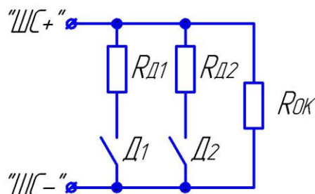
Рис.6 Схема подключения проводных пожарных дымовых датчиков к шлейфу с типом =15 (D1, D2 – контакты пожарных дымовых датчиков; Rok – оконечный резистор номиналом 5,6 кОм \pm 5\% ; RD1, RD2 – добавочные резисторы номиналом 2,2 кОм \pm 5\% . Максимальное допустимое сопротивление проводов шлейфа в данной схеме – 470 Ом; минимальное допустимое сопротивление утечки между проводами шлейфа – 7 кОм; максимальный допустимый ток утечки – 1,5 мА).
