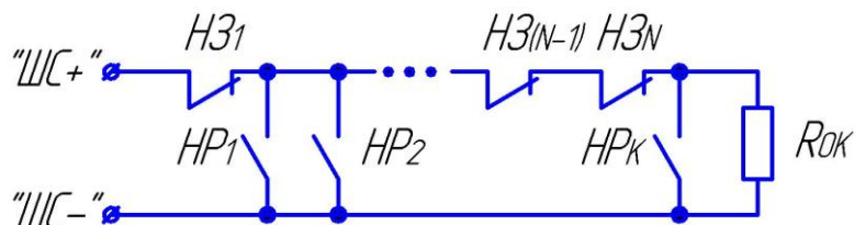
Рис.2 Схема подключения проводных охранных датчиков (НЗ – нормально замкнутый контакт охранного датчика; НР – нормально разомкнутый контакт охранного датчика; Rок – окончательный резистор номиналом 4,7 кОм \pm 5\% . Максимальное допустимое сопротивление проводов шлейфа в данной схеме – 470 Ом; минимальное допустимое сопротивление утечки между проводами шлейфа – 18 кОм; максимальный допустимый ток утечки – 0,6 мА).
