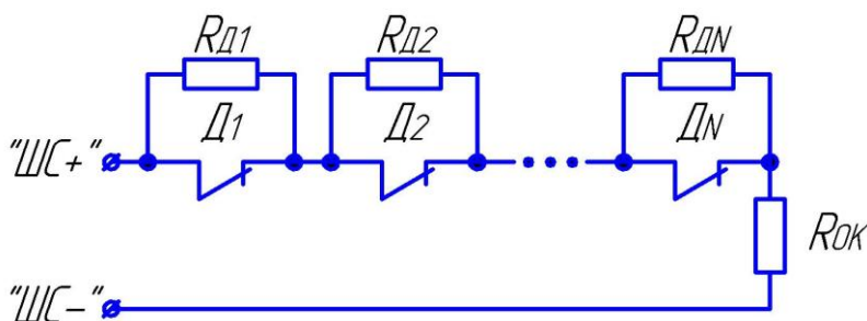
Рис.3 Схема подключения проводных пожарных тепловых датчиков к шлейфу с типом =7 (Д1...ДN – контакты пожарных тепловых датчиков; Rок – оконечный резистор номиналом 5,6 кОм ±5%; RД1, RД2 ... RДN – добавочные резисторы номиналом 5,6 кОм ±5%. Максимальное допустимое сопротивление проводов шлейфа в данной схеме – 470 Ом; минимальное допустимое сопротивление утечки между проводами шлейфа – 25 кОм; максимальный допустимый ток утечки – 0,4 мА).
