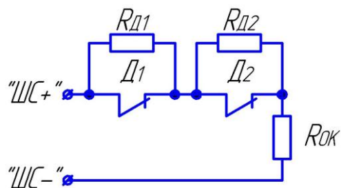
Рис.5 Схема подключения проводных пожарных тепловых датчиков к шлейфу с типом =15 (D1, D2 – контакты пожарных тепловых датчиков; Rok – оконечный резистор номиналом 4,3 кОм \pm 5\% ; RD1, RD2 – добавочные резисторы номиналом 6,8 кОм \pm 5\% . Максимальное допустимое сопротивление проводов шлейфа в данной схеме – 470 Ом; минимальное допустимое сопротивление утечки между проводами шлейфа – 50 кОм; максимальный допустимый ток утечки – 0,21 мА).
