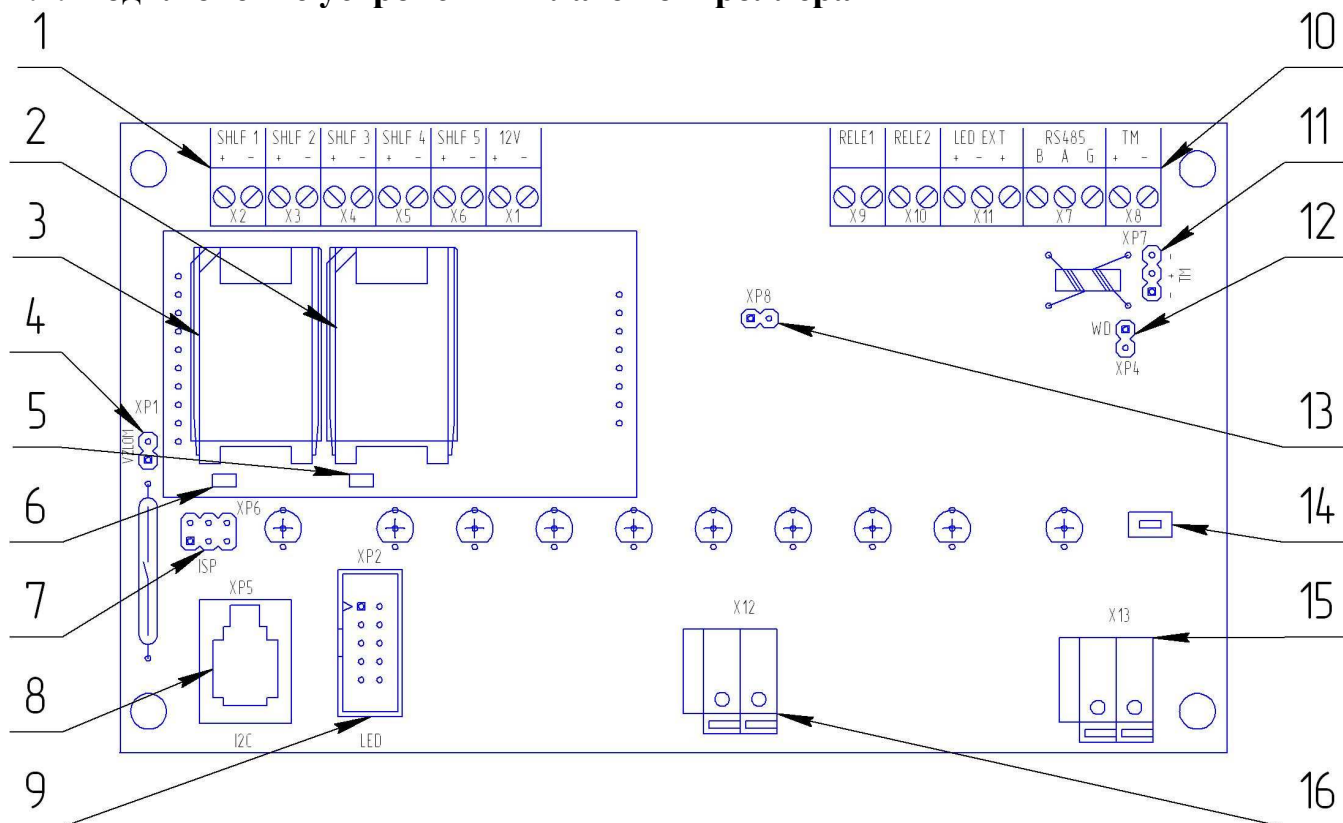
Рис.9 Внешний вид платы контроллера.
