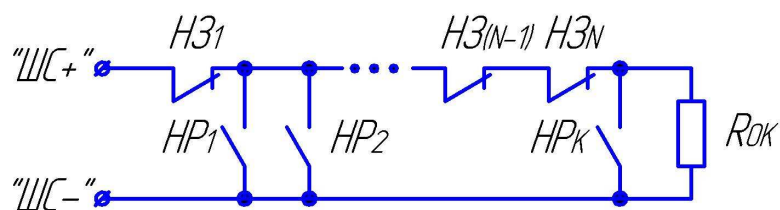
Рис.2 Схема подключения охранных датчиков (H3 – нормально замкнутый контакт охранного датчика; HP – нормально разомкнутый контакт охранного датчика; Rок – оконечный резистор номиналом 4,7 кОм ±5%. Максимальное допустимое сопротивление проводов шлейфа в данной схеме – 470 Ом; минимальное допустимое сопротивление утечки между проводами шлейфа – 18 кОм; максимальный допустимый ток утечки – 0,6 мА).
