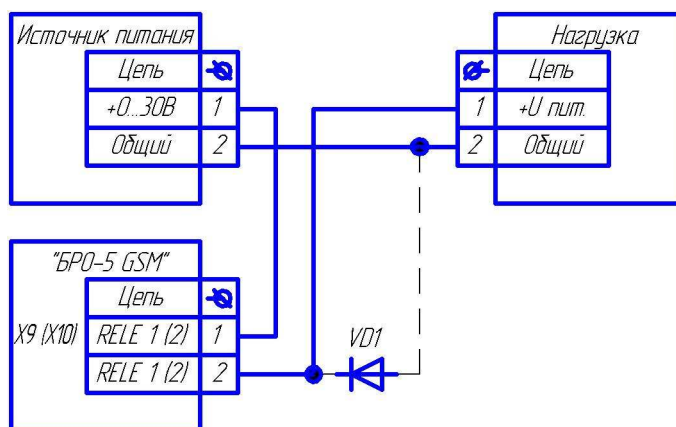
Рис.8 Подключение выходов при использовании отдельного источника питания (Напряжение на нагрузке 0...30В, максимальный ток потребления 120мА. Диод VD1 нужен, если нагрузкой является катушка реле. Допустимое обратное напряжение диода должно превышать напряжения источника питания)
