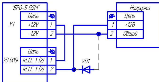
Рис.7 Подключение выходов при использовании встроенного в блок источника питания (Напряжение на нагрузке 10,5...13,7В, максимальный ток потребления 100мА. Диод VD1 нужен, если нагрузкой является катушка реле. Допустимое обратное напряжение диода должно быть не менее 20В)
