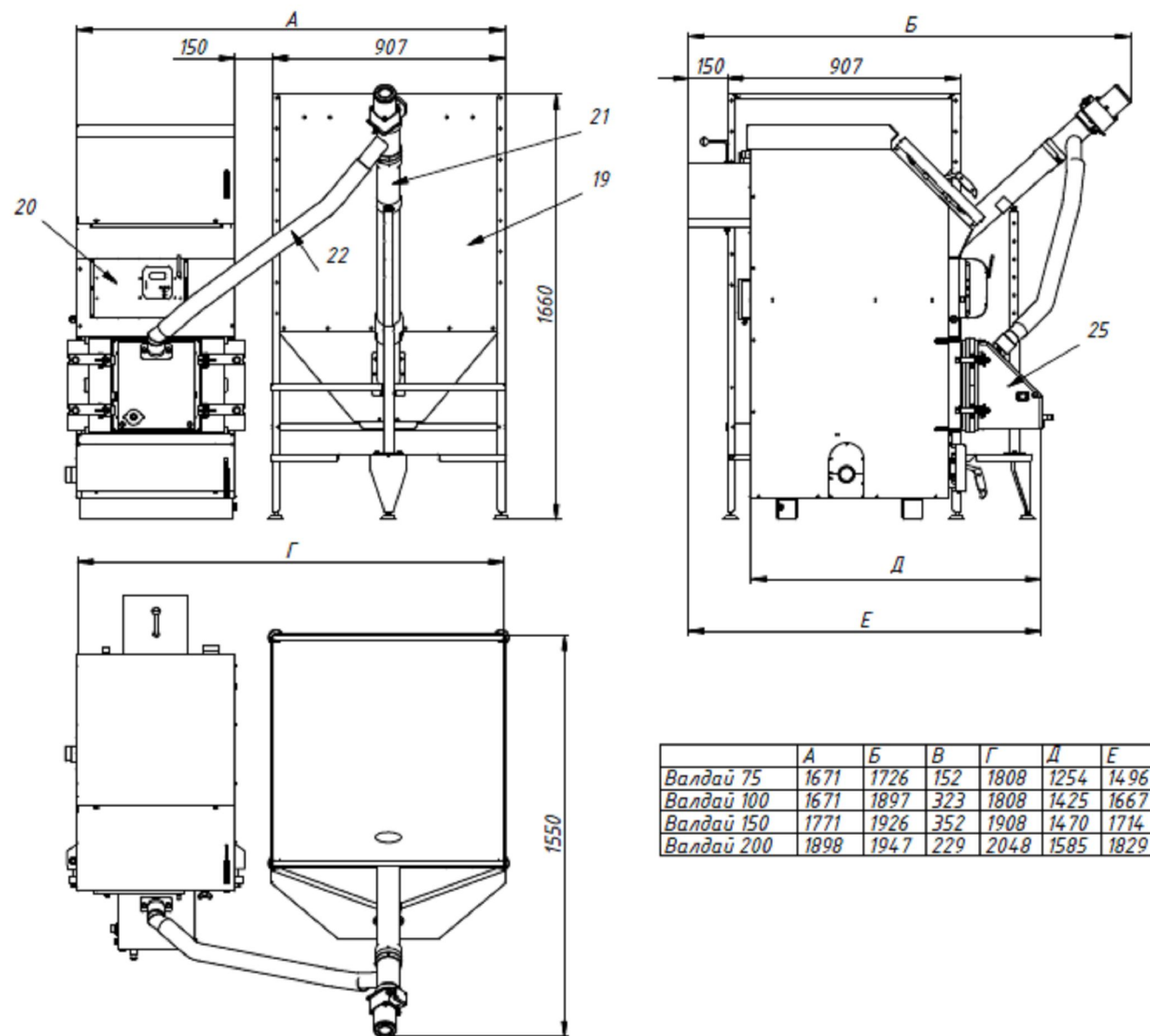
Рис. 2. Компонировка котла с бункером.
