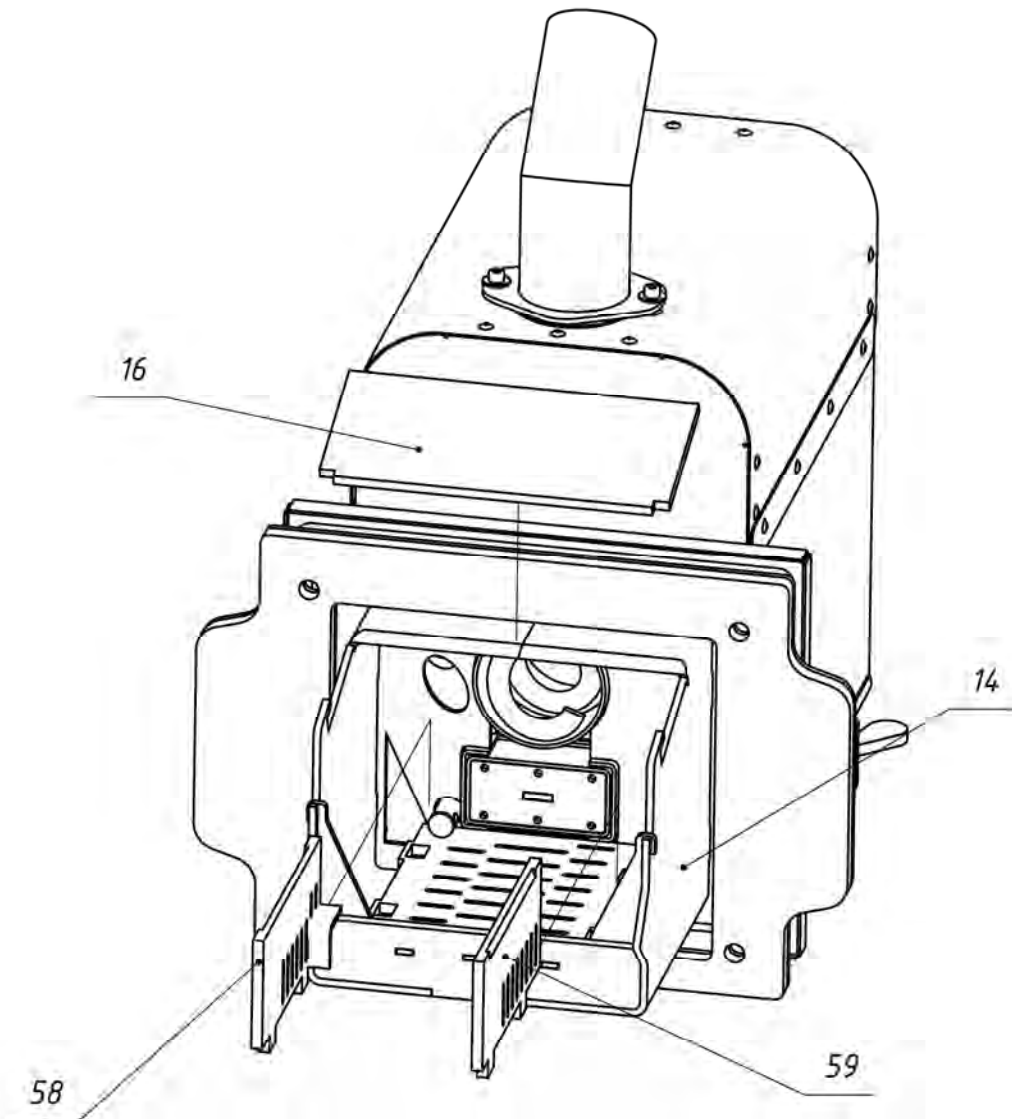
Рис. 78 Вынуть из камеры сгорания боковины колосника (поз. 58 и 59).
