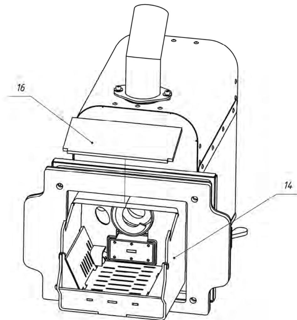
Рис. 7а Снять крышку камеры сгорания горелки.
