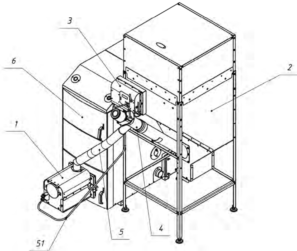
Рис. 16 Размещение горелки на котле.
