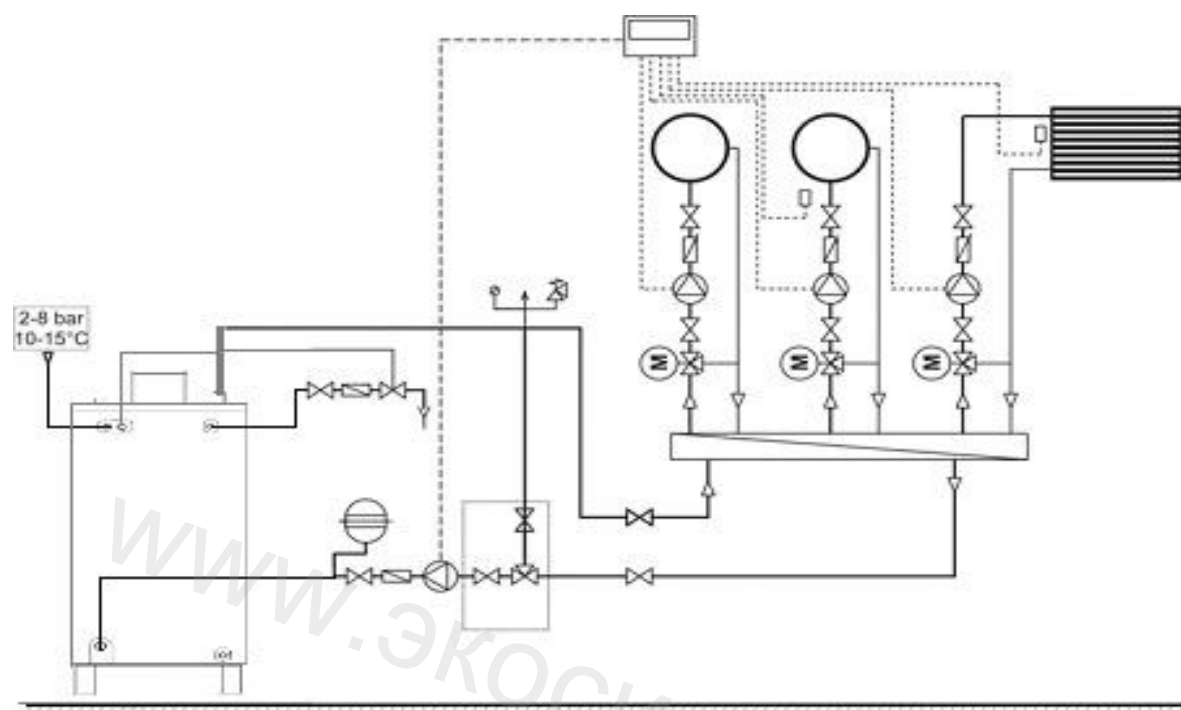
Диаграмма 7. Подключение котла BW LIGHT с трехходовым клапаном
