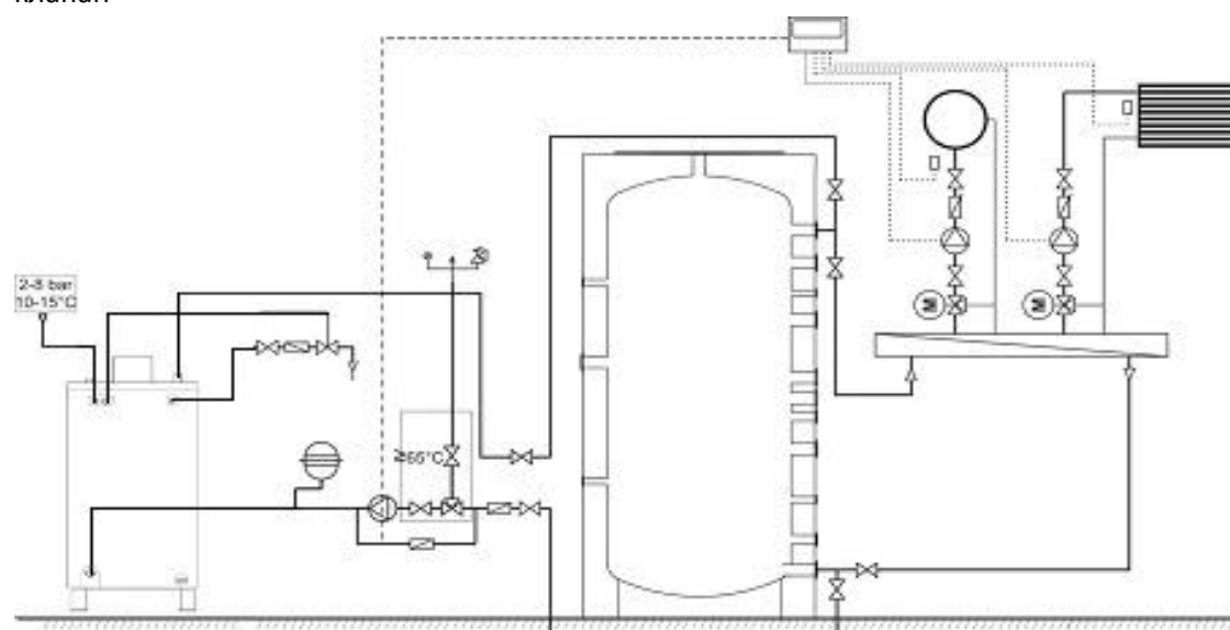
Диаграмма 8. Подключение котла BWLIGHT типа BA буферный резервуар и трехходовой клапан
