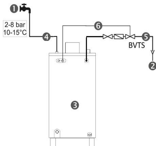
Диаграмма 6. Подключение теплообменника безопасности тепла
