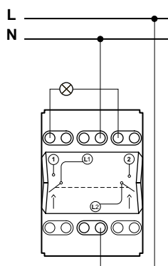
Двухполюсный переключатель
