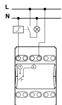
Кнопочный выключатель
