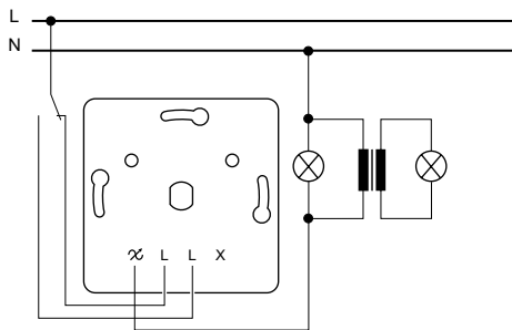
Переключатель – S5xx511-S5xx518
