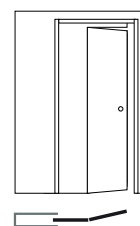
ECLISSE NOVANTA 56 - 57
