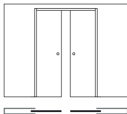
ECLISSE DOUBLE 24 - 25
