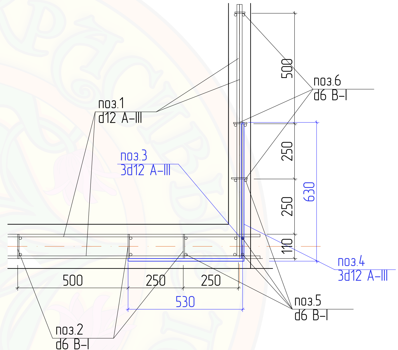
Узел 2 М 1:10
