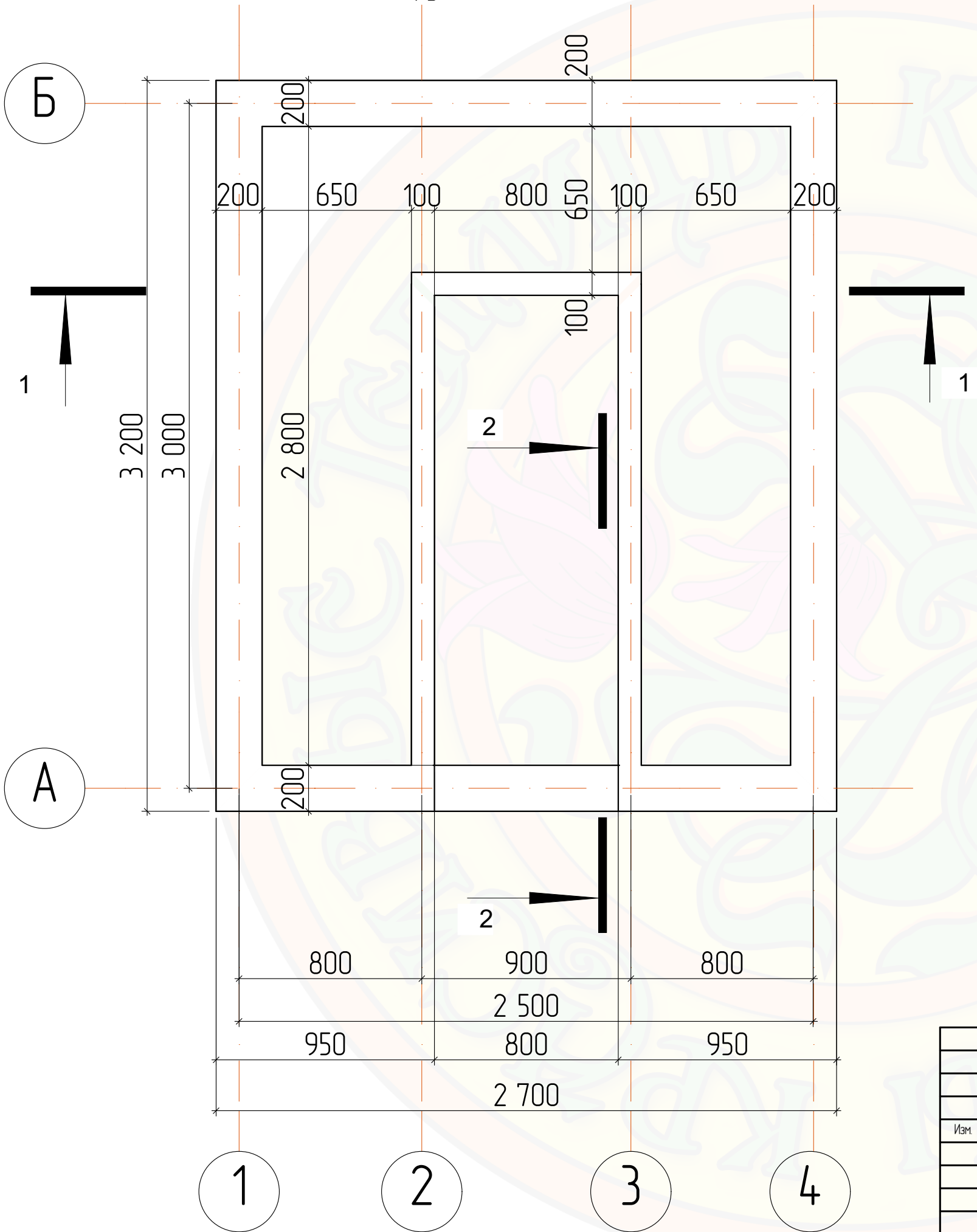
План фундамента М 1:20
