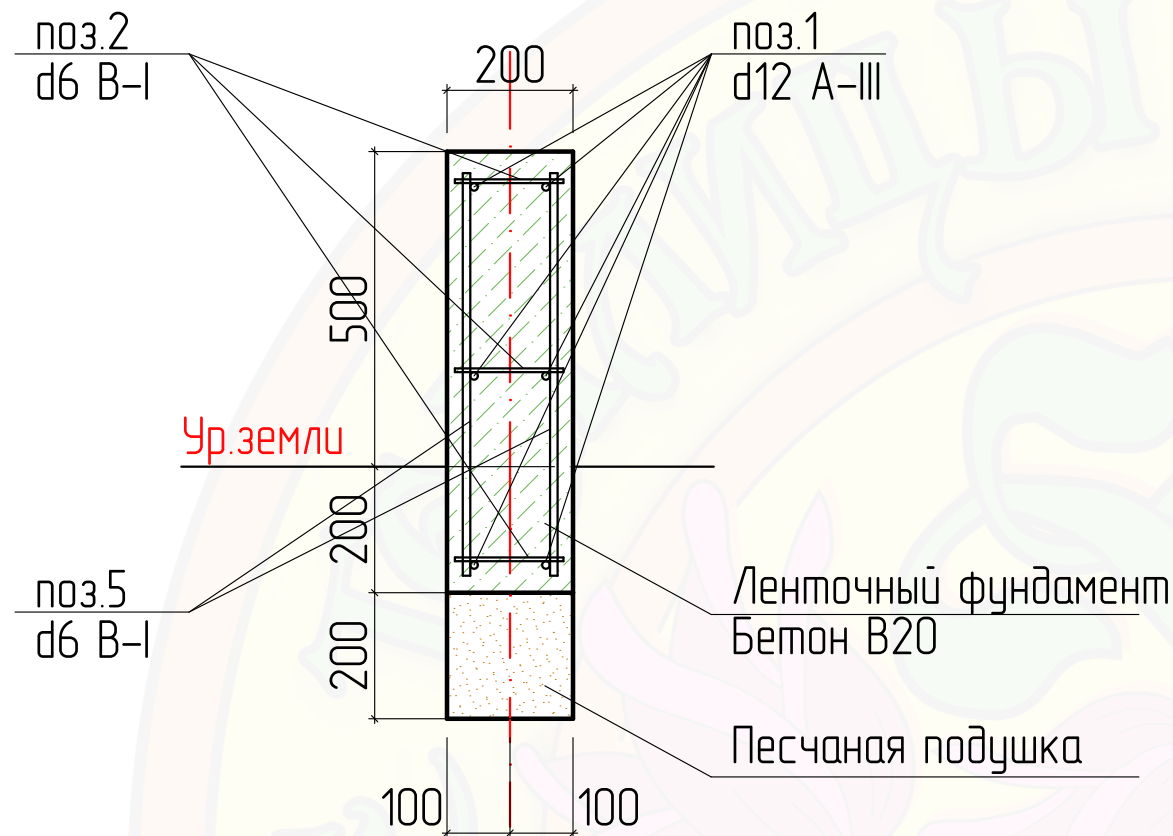
Узел 3 М 1:10
