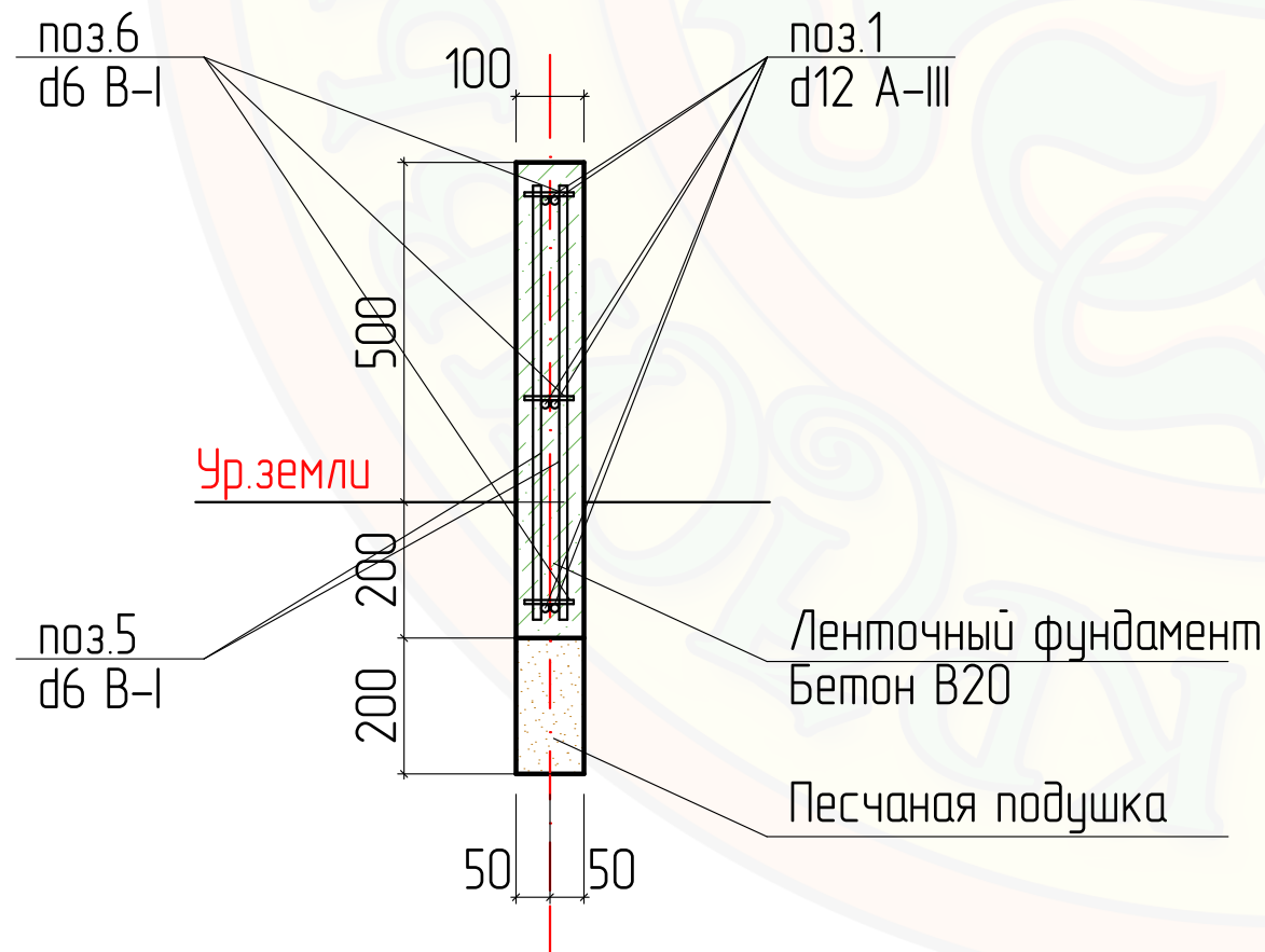
Узел 4 М 1:10
