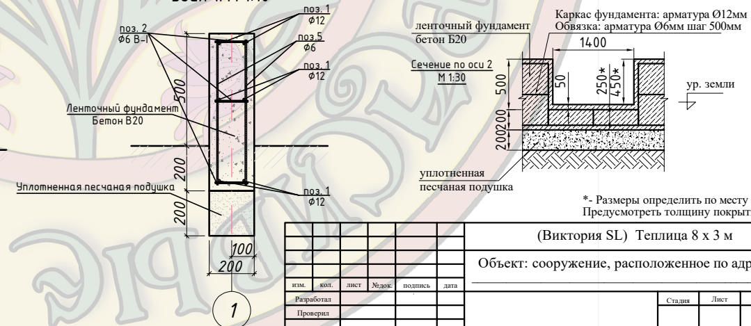
Узел 1. М 1:10
