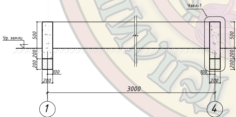
Разрез 1-1. М 1:40
