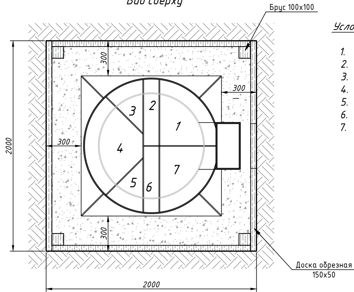
Вид сверху
