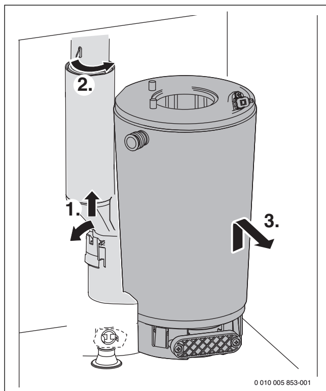
Рис. 66 Демонтаж теплообменника
