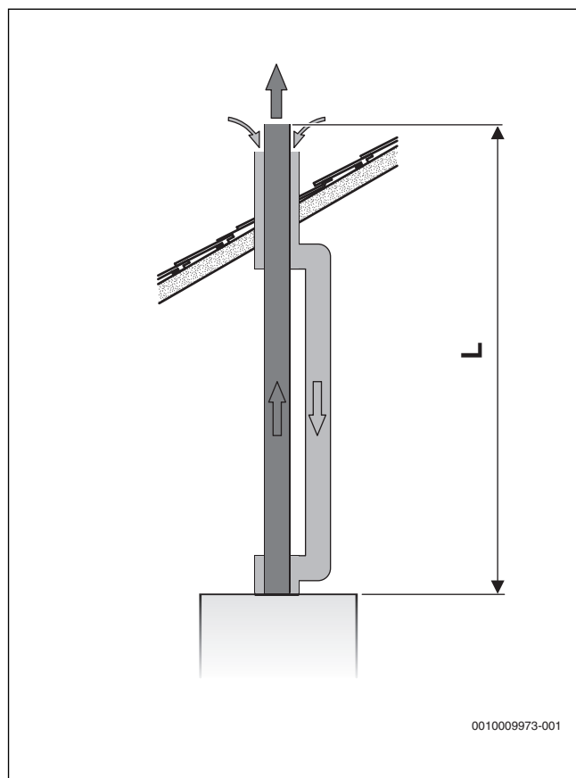
Рис. 15 Вертикальный отвод дымовых газов по C_{33(x)}
