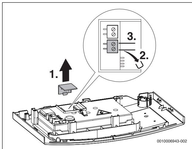
Рис. 28 Подключение регулятора
