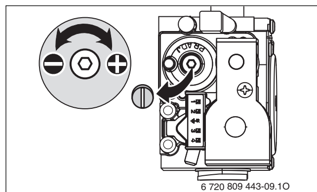
Рис. 38 Удаление пломбы с газовой арматуры
