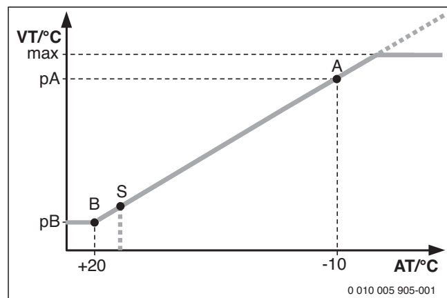
Рис. 68 Отопительная кривая
