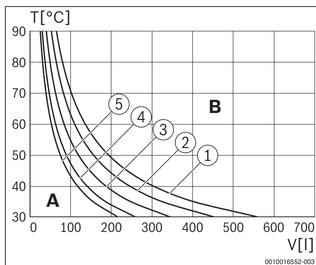
Рис. 22 Характеристики расширительного бака
