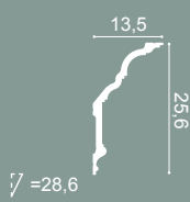
C340 200 x 25,6 x 13,5 cm Purotouch®
