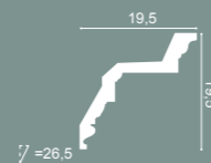
1 C307 + C307A 2 C307A: 7,5 x 4 x 9,4 Duropolymer®
