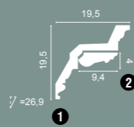
1 C307 + C307A 2 C307A: 7,5 x 4 x 9,4 Duropolymer®
