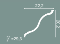
C335 200 x 22,2 x 20,2 cm Purotouch®
