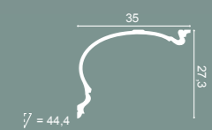
C344 HERITAGE XXL 200 x 27,3 x 35 cm Purotouch®
