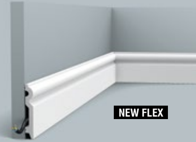
SX137 | SX137F 200 x 9,9 x 1,5 cm Duropolymer ®
