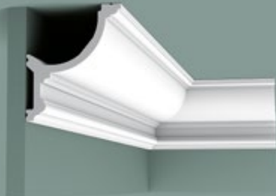
C901 | C901F 200 x 14,8 x 12,4 cm Purotouch ® 12,4 14,8 17 = 19,2
