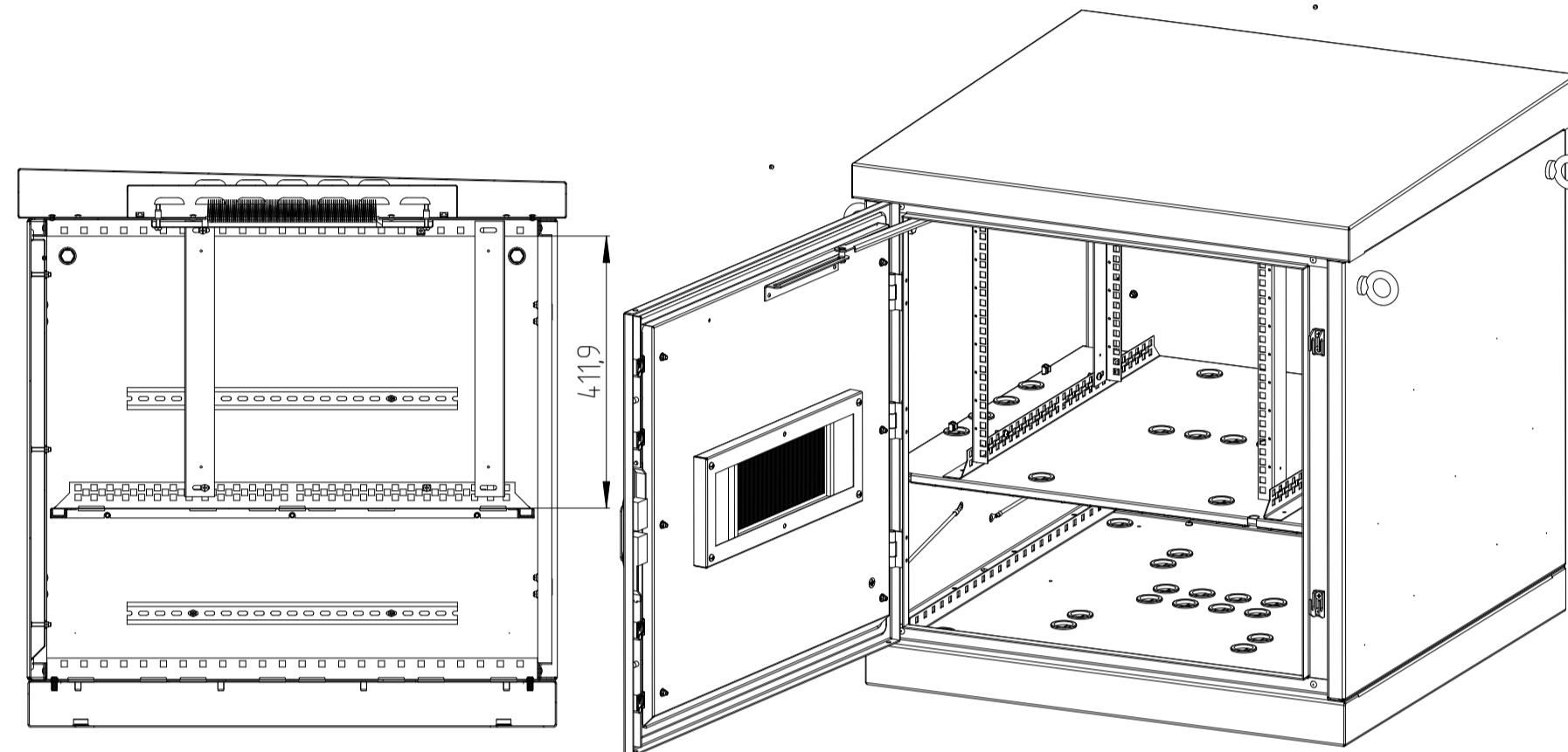
ШТВ-1-9U.8.8-4AAA
