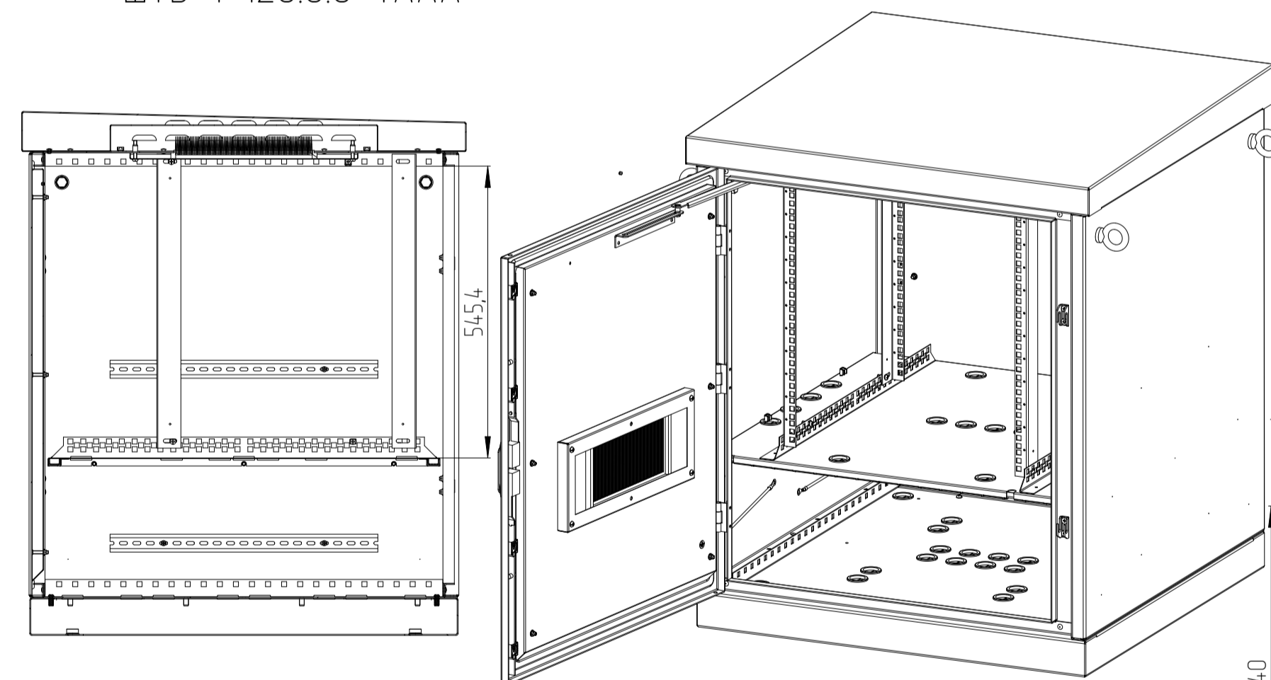
ШТВ-1-12U.8.8-4AAA
