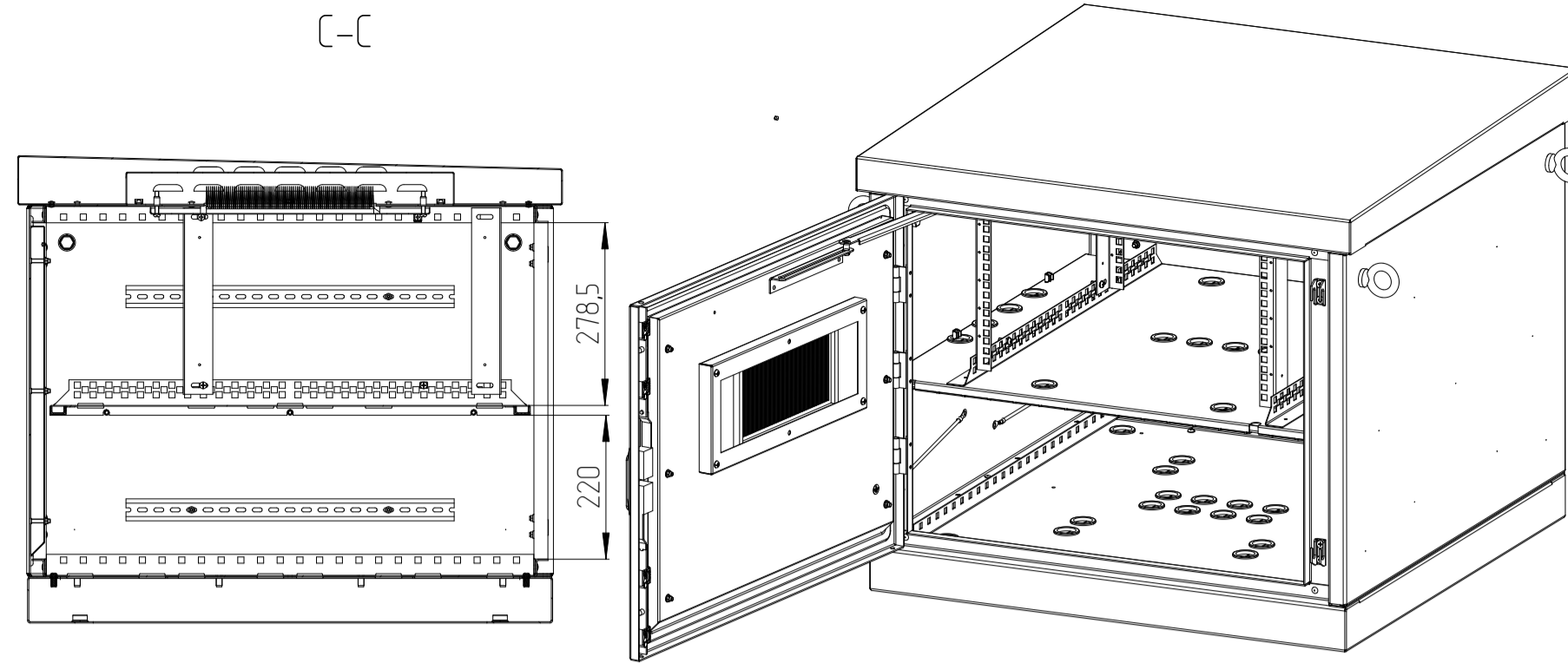
ШТВ-1-6U.8.8-4AAA
