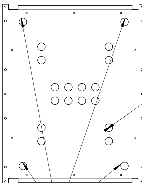
Основа каркаса ШТВ-1-х6.8
