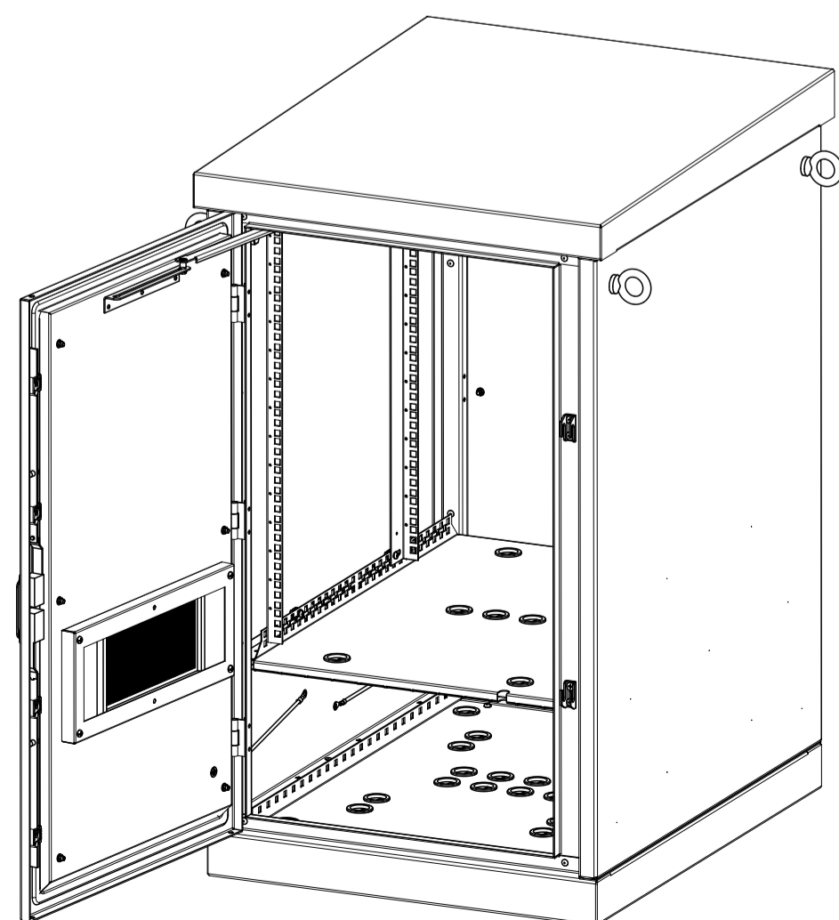
Основа каркаса ШТВ-1-х6.8
