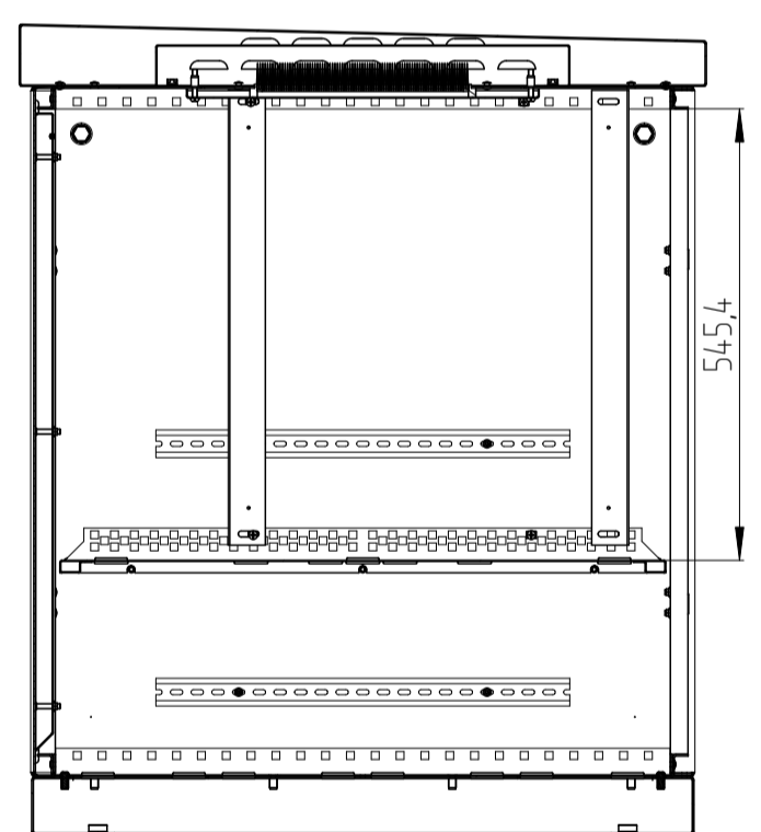
ШТВ-1-15U.6.8-4AAA
