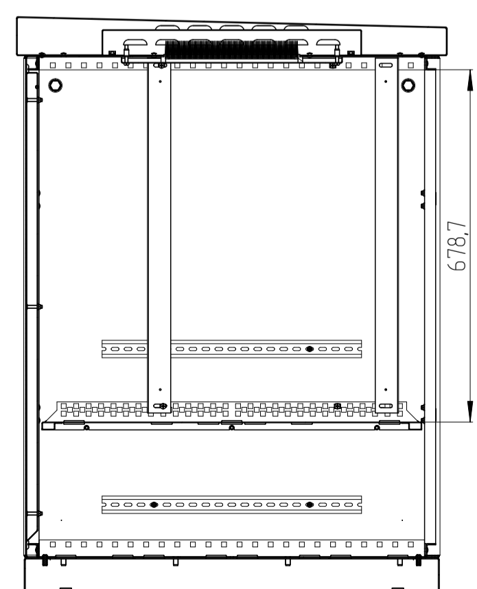
ШТВ-1-15U.6.8-4AAA
