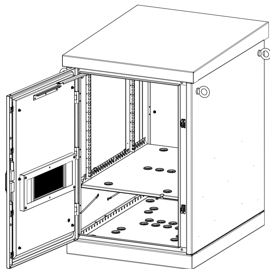
Основа шкафа ШТВ-1-х6.8
