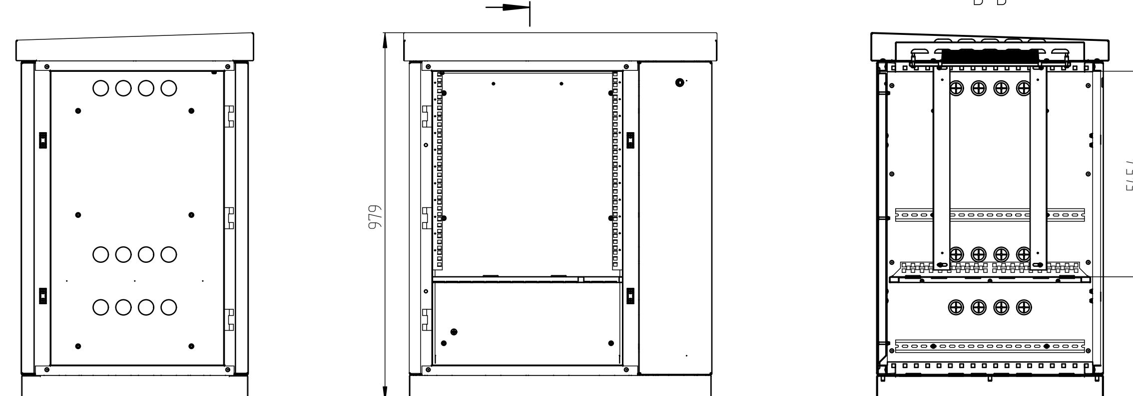
ШТВ-2-15U.8.6-4AA3
