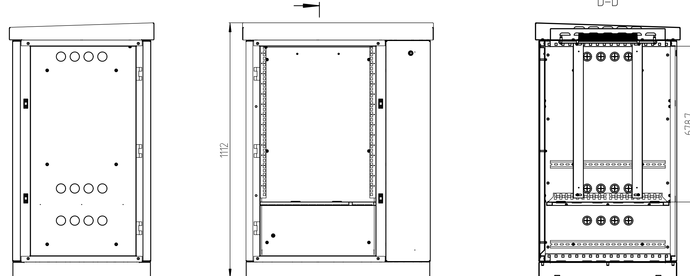
ШТВ-2-18U.8.6-4AA3
