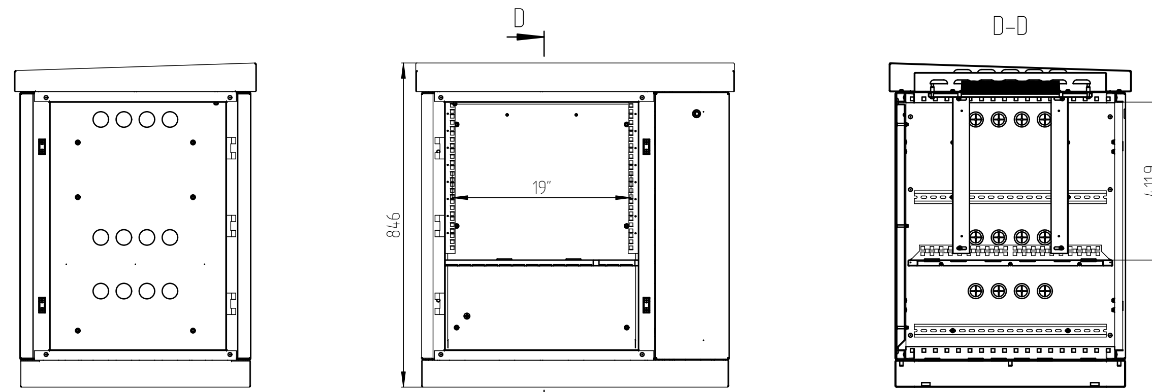
ШТВ-2-12U.8.6-4AA3
