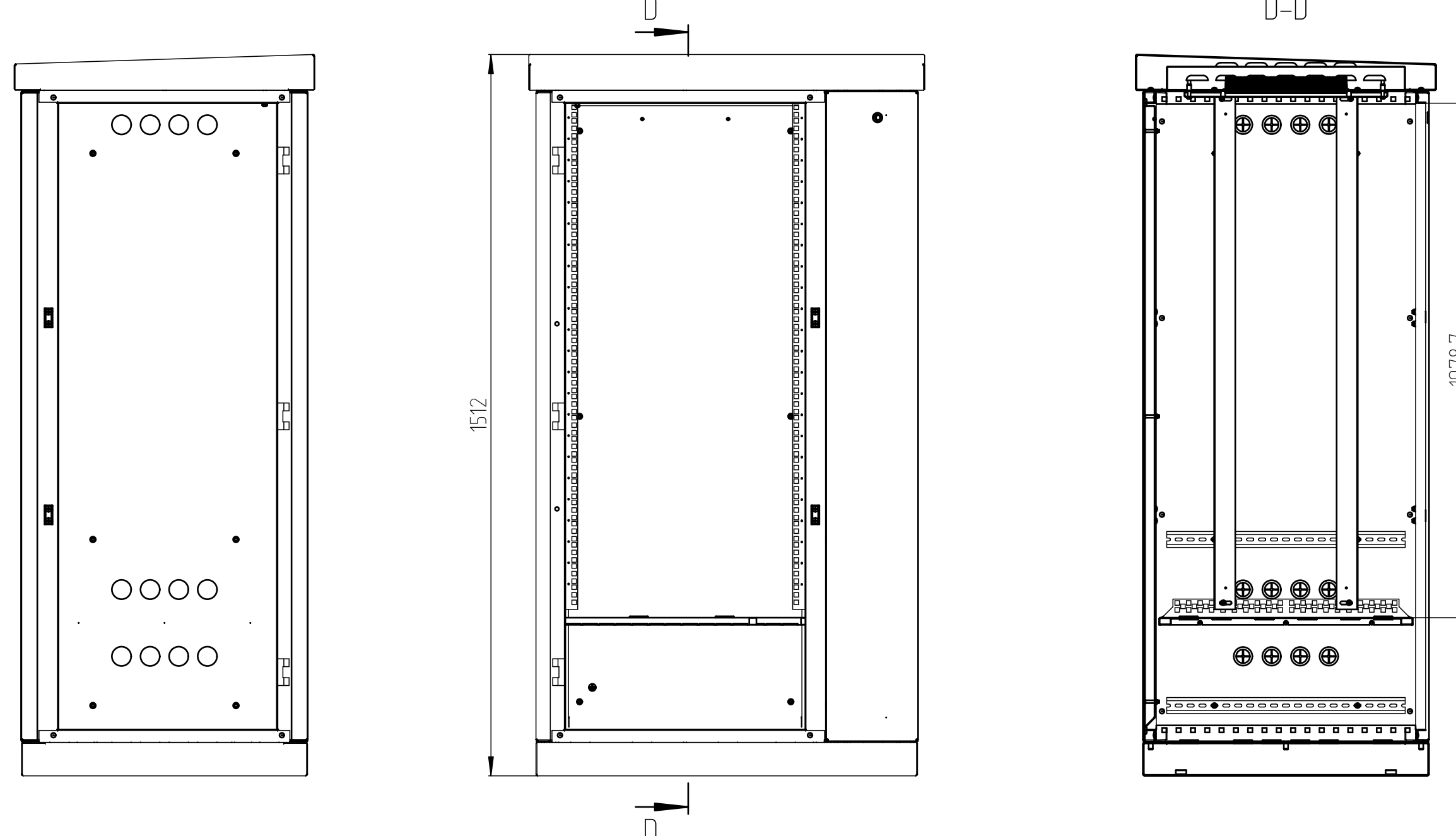
ШТВ-2-24U.8.6-4AA3
