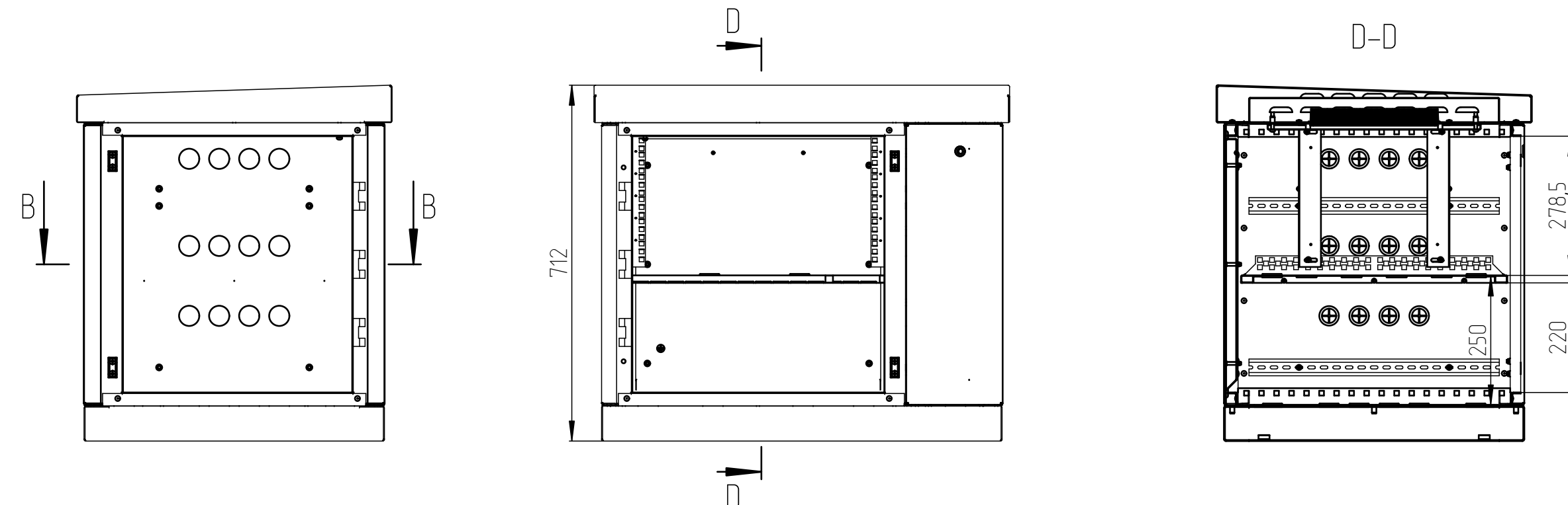
ШТВ-2-9U.8.6-4AA3
