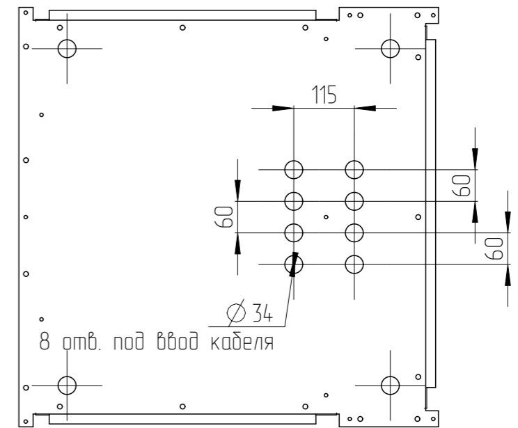
Основание каркаса
