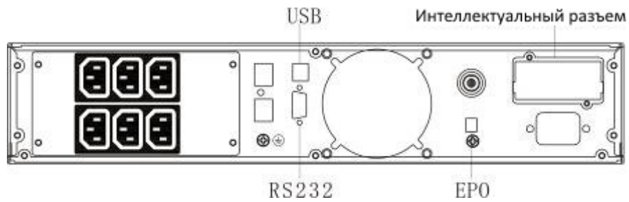
Рис. 20. Настройки коммуникации и терминалы управления (показана модель Rack/Tower 1кВА)
