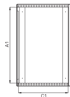
Вид сбоку (внутренняя часть)
