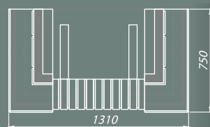
ОБЛИЦОВКА ПРИСТЕННАЯ С КАМЕННОЙ БАЛКОЙ
