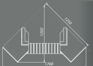
ОБЛИЦОВКА УГЛОВАЯ С ДЕРЕВЯННОЙ БАЛКОЙ
