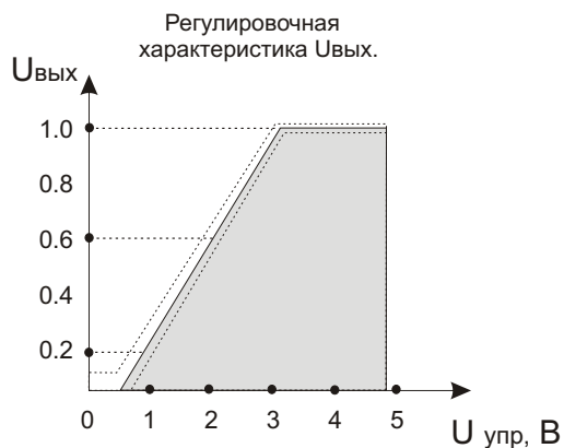
Типовая выходная характеристика
