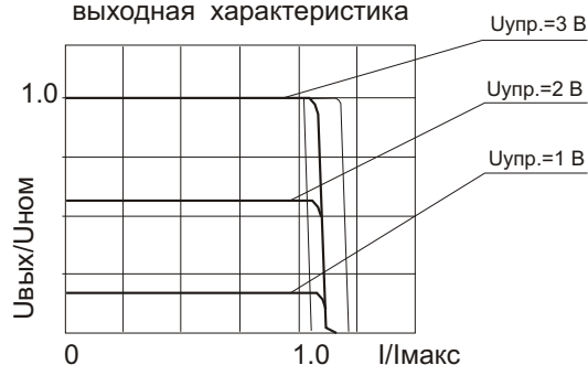
Типовая выходная характеристика
