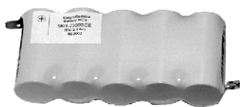
Рис.5 Образец сборки из Ni-CD и Ni-MH элементов.
