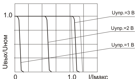
Типовая выходная характеристика
