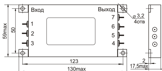
Габаритные размеры
