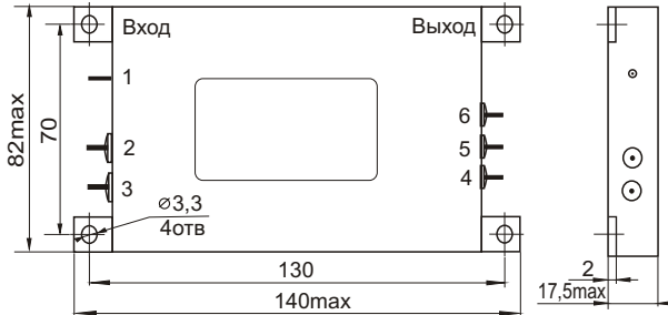
Габаритные размеры
