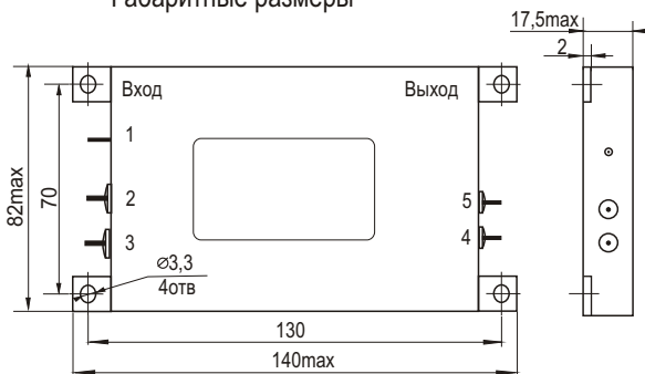
Габаритные размеры
