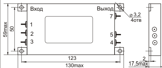
Габаритные размеры
