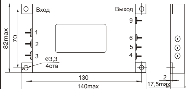
Габаритные размеры
