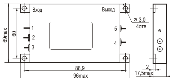
Габаритные размеры
