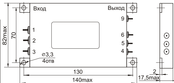
Габаритные размеры
