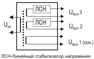
ЛСН-Линейный стабилизатор напряжения
