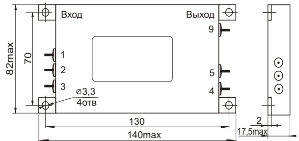
Габаритные размеры для блоков мощностью 50(60)Ватт кроме изделий с выходным напряжением до 9 Вольт
