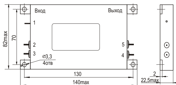
Габаритные размеры
