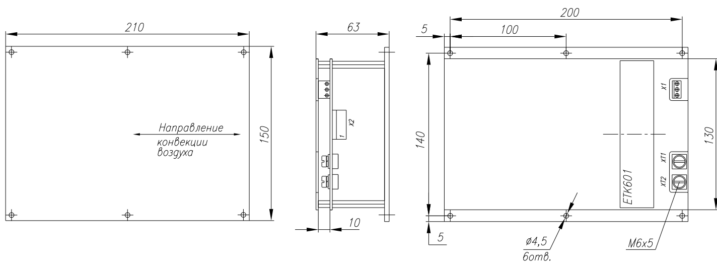
Рис.11 Корпус ТК601
