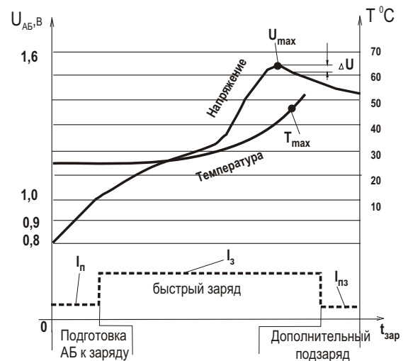
Рис.1 Временная характеристика заряда
