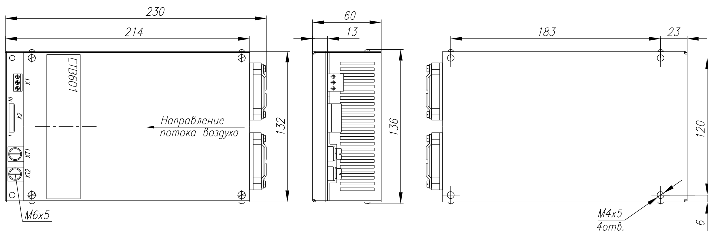
Рис.10 Корпус ТВ601
