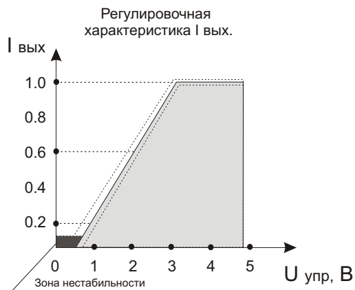
Типовая выходная характеристика
