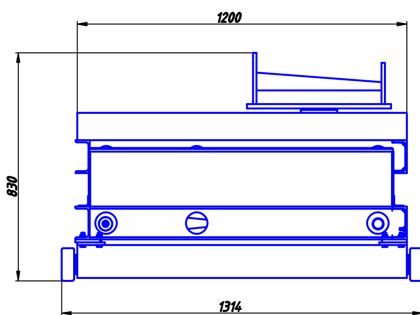
Подъёмник сложен
