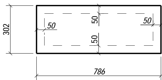
GB031 - 2 шт.
