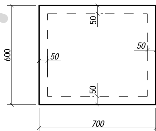
GB029 - 18 шт.
