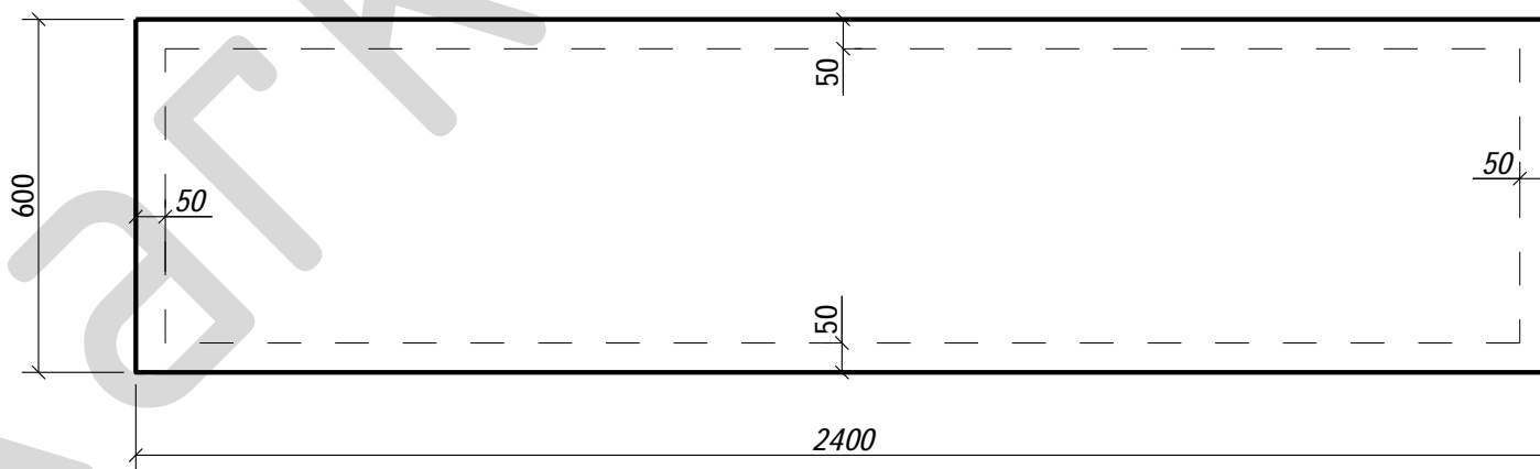
GB033 - 1 шт.
