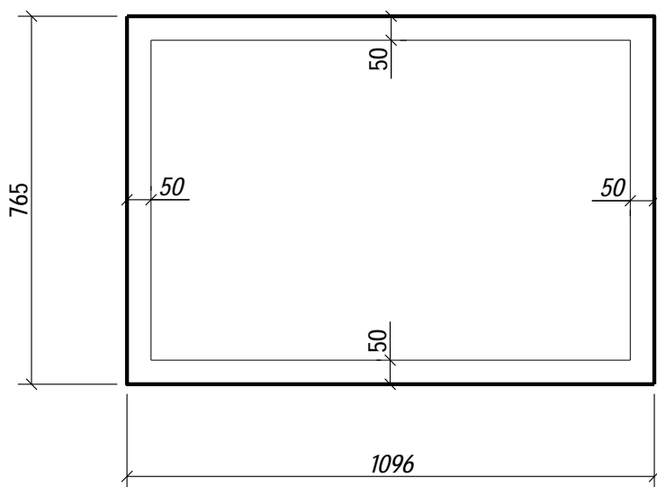
S041 - 1 шт.
