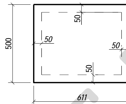
S036 - 1 шт.
