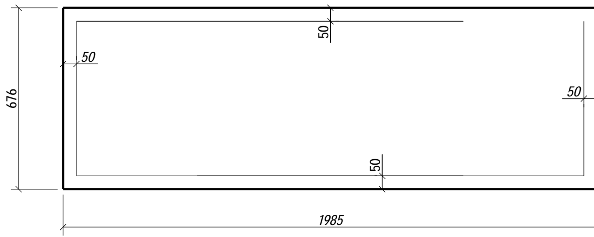
S028 - 1 шт.
