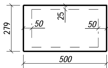
S042 - 1 шт.
