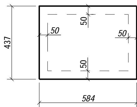
GB003 - 3 шт.
