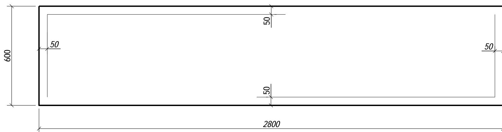
GB001 - 32 шт.
