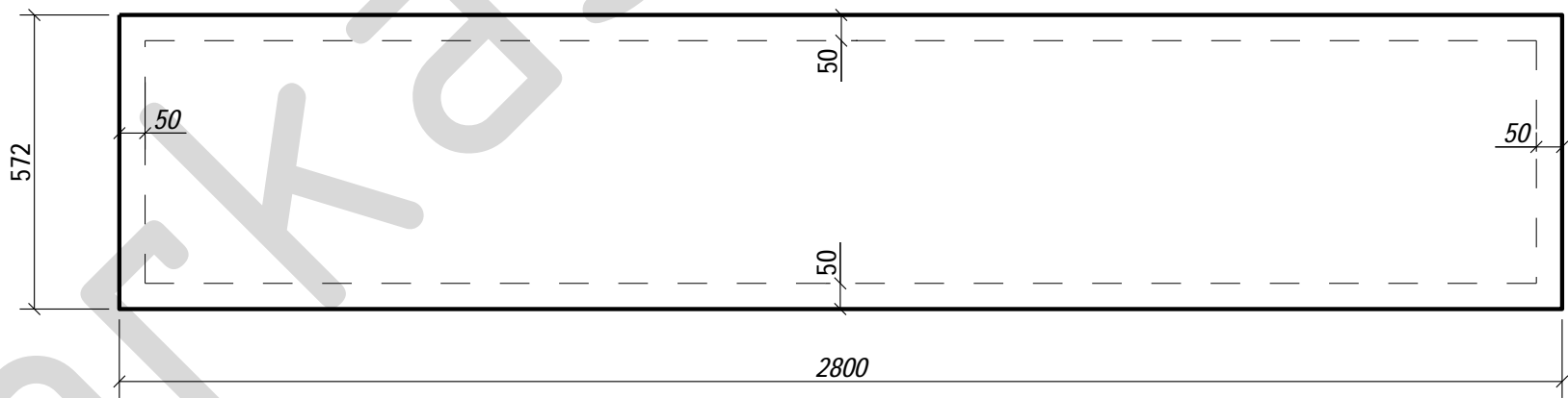
GB018 - 3 шт.
