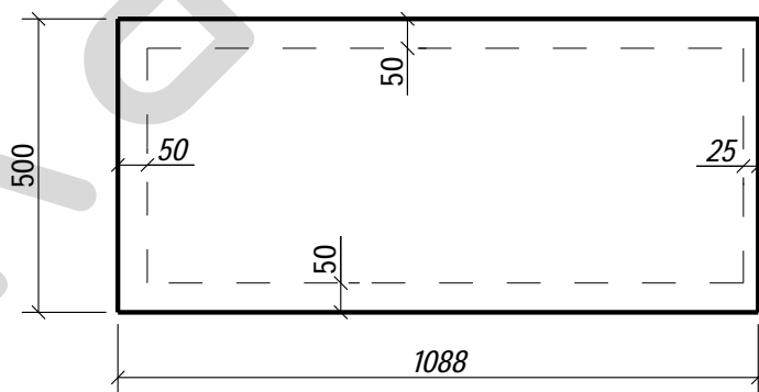
S004 - 1 шт.
