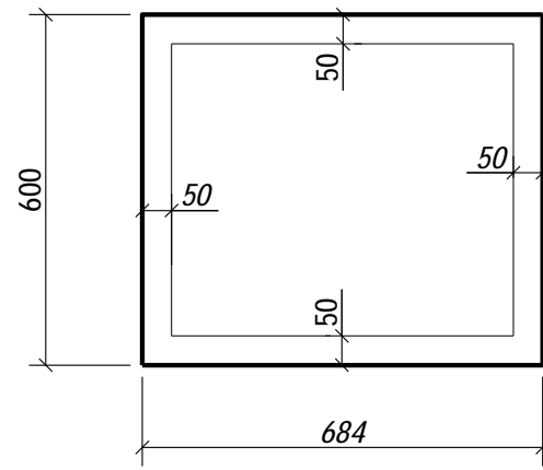
GB011 - 1 шт.
