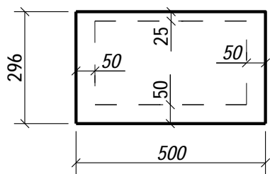
S040 - 2 шт.
