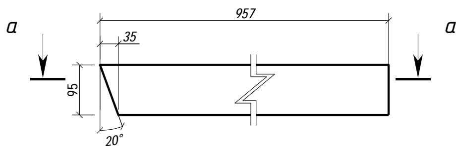
Д068 - 2 шт.
