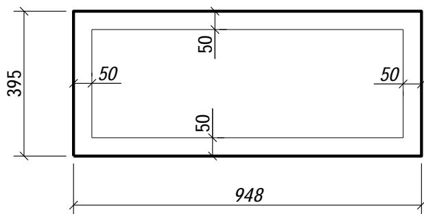
S001 - 2 шт.
