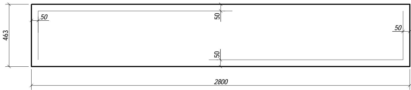
GB020 - 12 шт.
