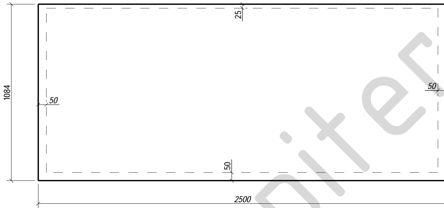
S029 - 1 шт.
