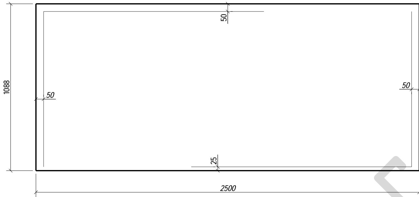
S005 - 1 шт.
