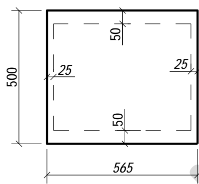
S050 - 1 шт.
