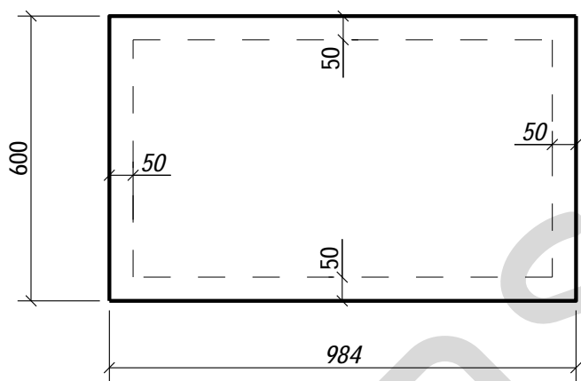
GB032 - 1 шт.
