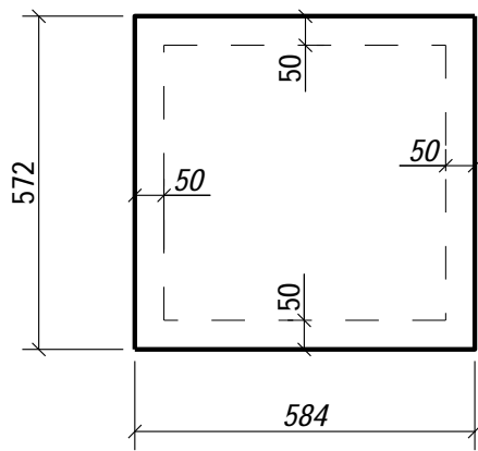
GB017 - 1 шт.
