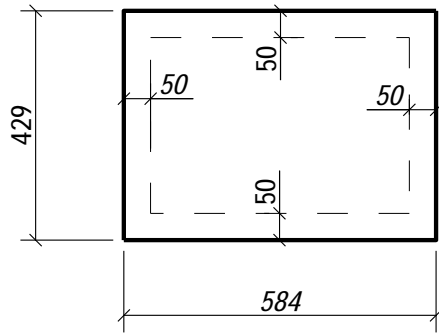
GB016 - 1 шт.
