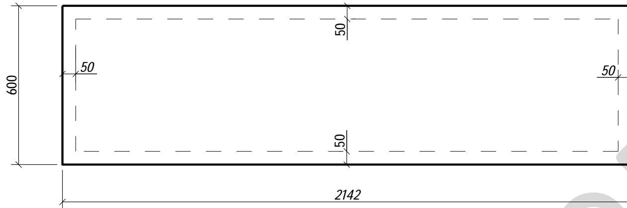
GB026 - 3 шт.
