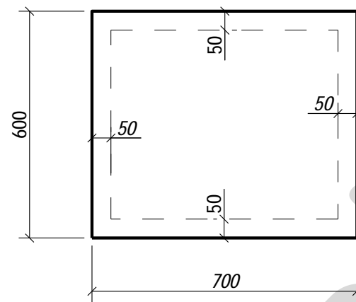
GB012 - 9 шт.
