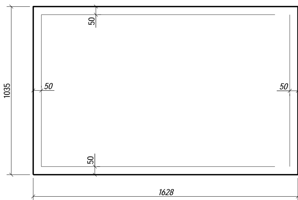
S016 - 2 шт.
