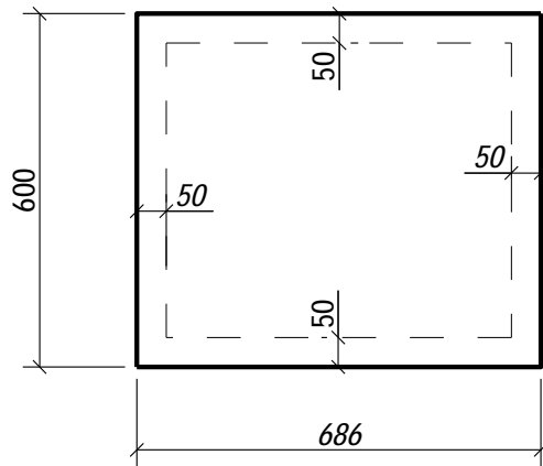
GB021 - 2 шт.
