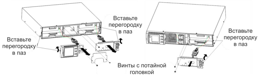
Рисунок 20 – Отсоединение перегородок
