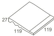
Duş parçası Shower inclined end edge M 12.5 x 12.5 cm / 5" x 5" 119 x 119 x 27 mm EN14411 B1b
