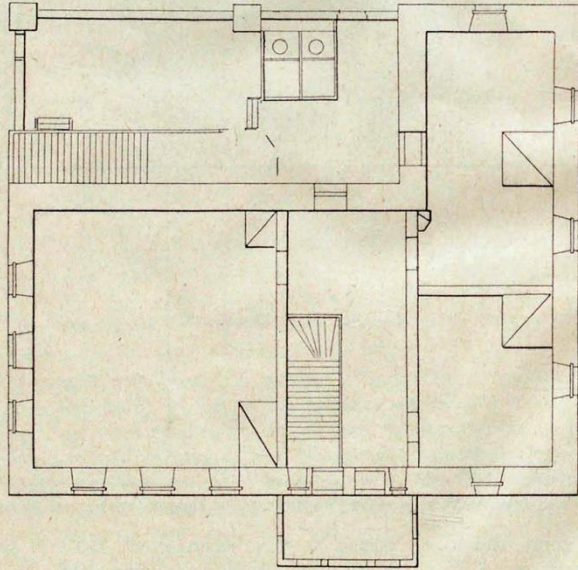
Планъ нижняго, богадельнаго, этажа и видъ церковнаго дома, въ которомъ помѣщается школа.
