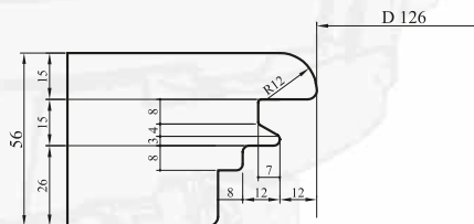
G 08 - PROFILO TRAVERSI E MONTANTI TELAIO
