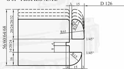
G 01 - PROFILO ANTE
