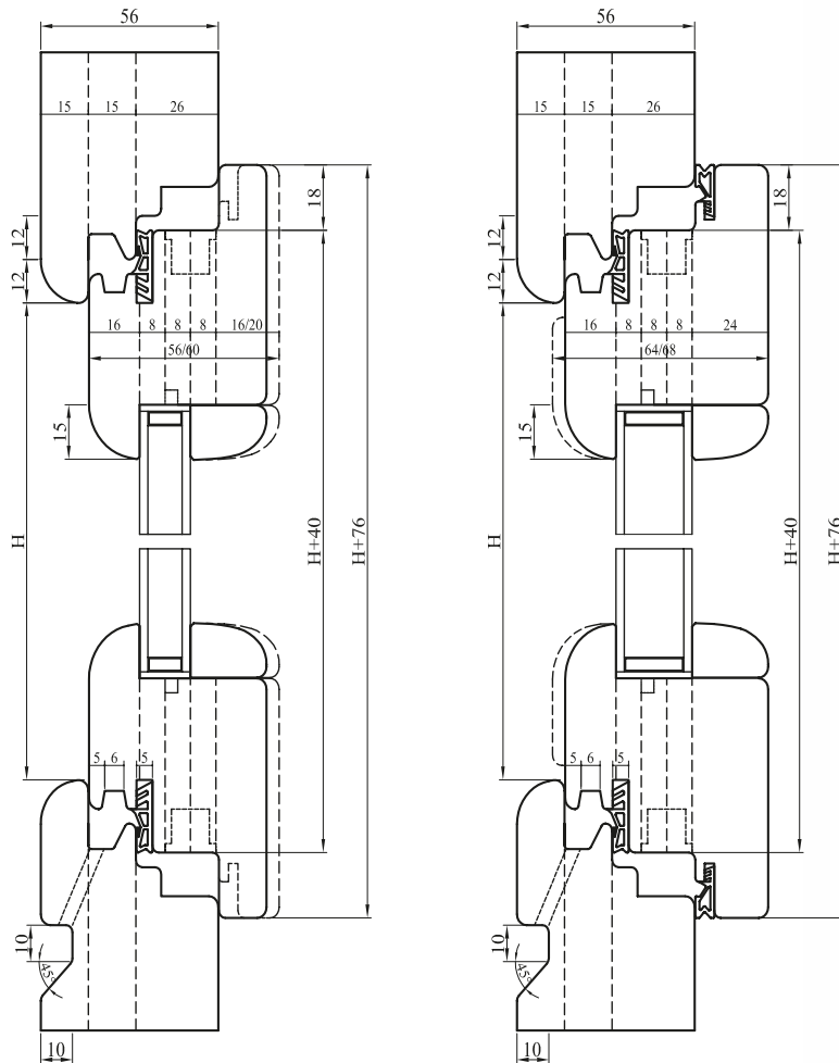
SEZIONE VERTICALE LEGNO 56 / 60 / 64 / 68 VERTICAL WOOD SECTION 56 / 60 / 64 / 68
