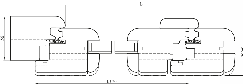
SEZIONE ORIZZONTALE LEGNO 56 / 60 / 64 / 68 HORIZONTAL WOOD SECTION 56 / 60 / 64 / 68
