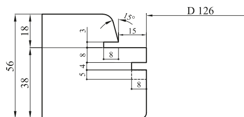
G 12 - PROFILO TRAVERSI INFERIORE TELAIO
