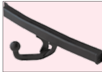
Тип шара «H» – сварной, грузоподъемность 1500 кг
