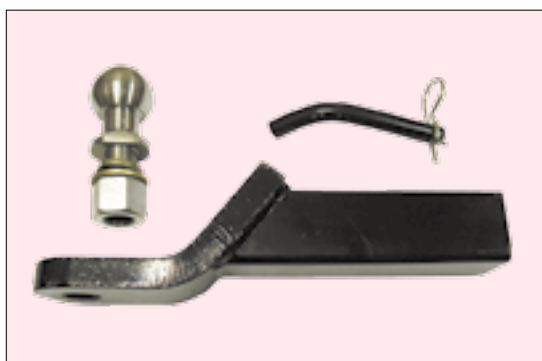
Шар для «американских» авто на базе шара «Е». Грузоподъёмность 1500кг. №VFM – 80-01E
