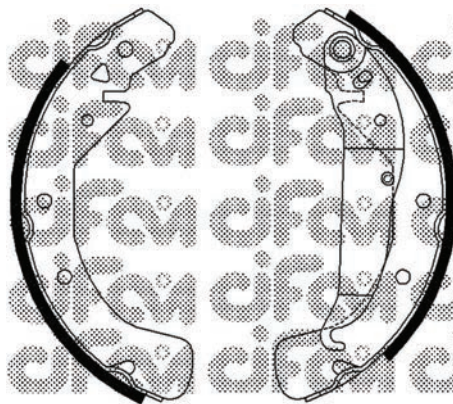
153-311 (Ø 230,0 x 42)
