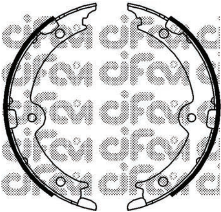
153-449 (Ø 190,0 x 26)
