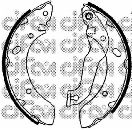
153-166 (Ø 203,2 x 39)
