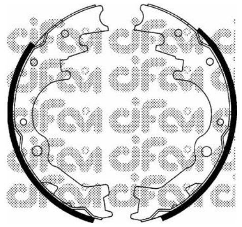
153-208 (Ø 260,0 x 50)
