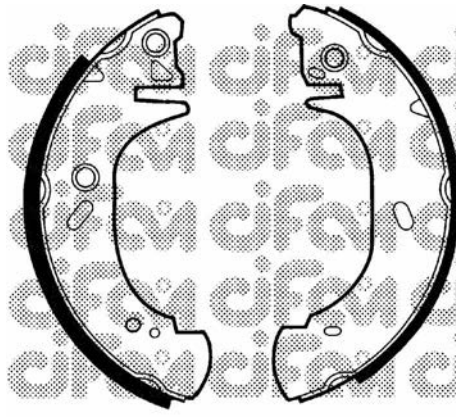
153-127 (Ø 280,0 x 64)
