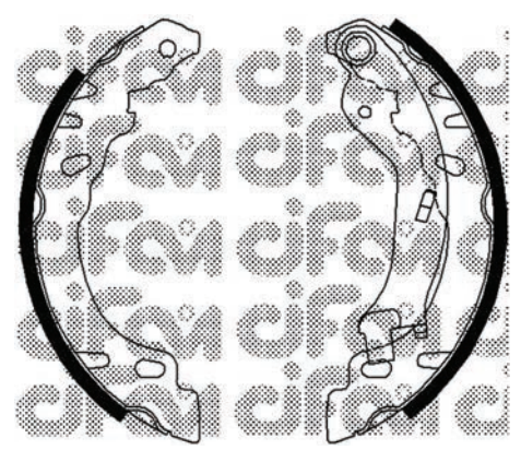
153-090 (Ø 180,0 x 30)
