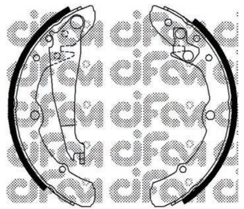
153-008 (Ø 230,0 x 40)
