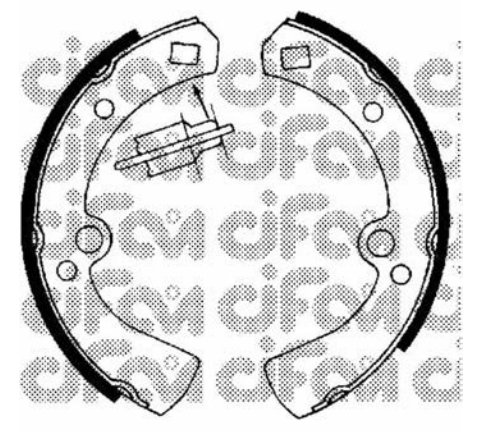
153-270 (Ø 203,2 x 36)
