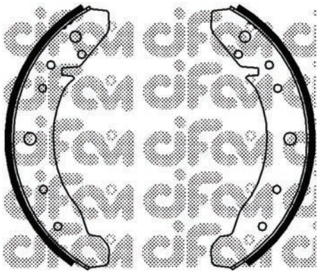
153-457 (Ø 230,0 x 40)
