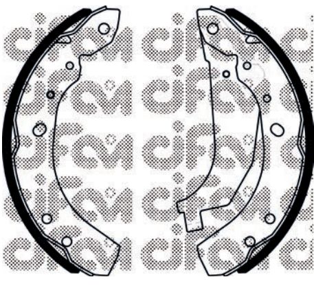
153-482 (Ø 220 x 42)
