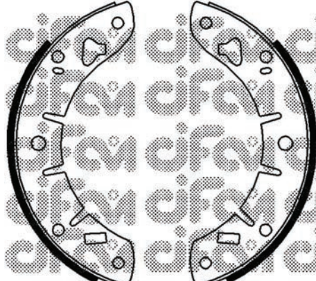
153-007 (Ø 254,0 x 45)
