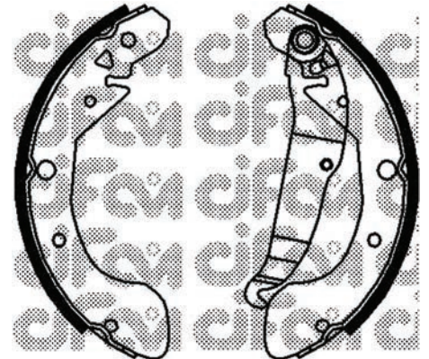
153-049 (Ø 230,0 x 52)
