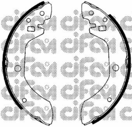
153-271 (Ø 228,6 x 40)
