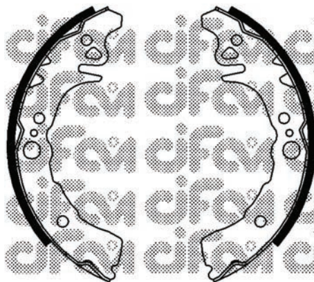
153-039 (Ø 180,0 x 38)
