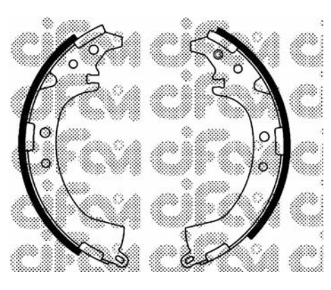
153-429 (Ø 228,6 x 42)
