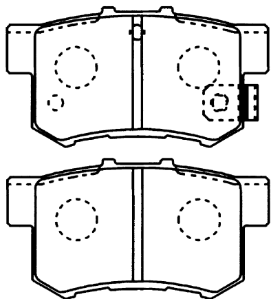
AN - 492WK アコード、S2000 (Rr)
