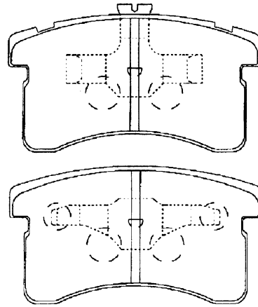
AN - 345K ミラ、クォーレ
