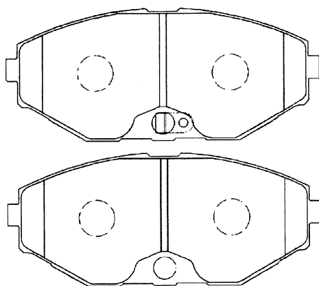
AN - 372WK セドリック、シーマ
