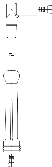
Anschluß Verteilerkappe/Zündspule: 4 mm, Toyota 5 mm, DIN
