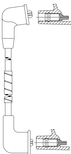
Anschluß Zündkerze: M4, SAE
