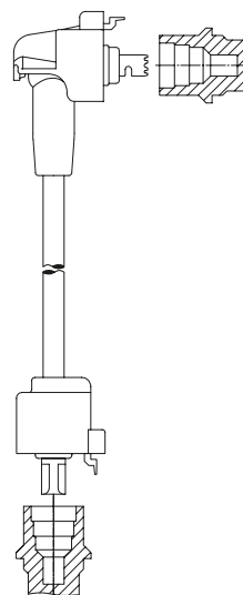
Anschluß Verteilerkappe/Zündspule: 4 mm, Toyota 5 mm, DIN
