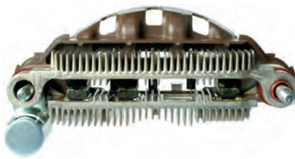
132714 Rectifier
