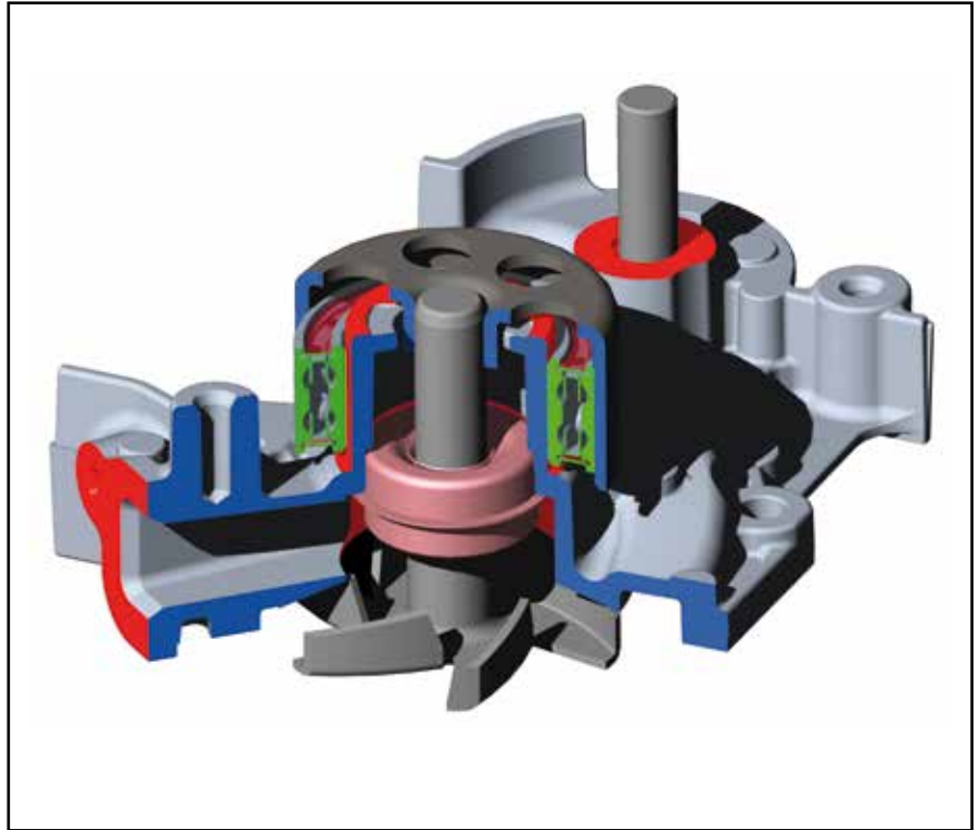
11.2 Modello 3D di pompa acqua con evidenziato in verde il cuscinetto esterno al corpo pompa
