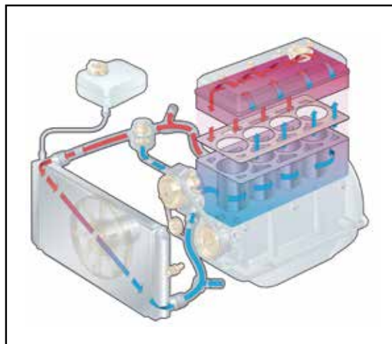
1.4 Schema moderno circuito di raffreddamento
