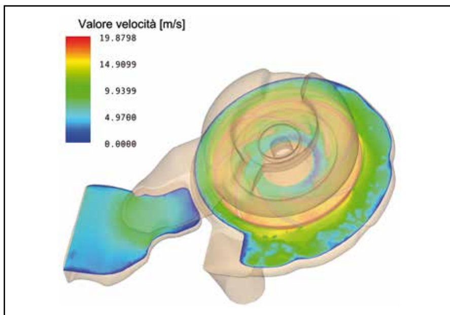
6.1 Analisi fluidodinamica di una pompa acqua
