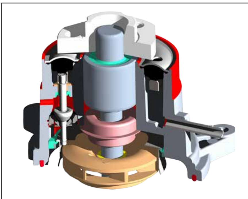
12.1 Sezione della pompa acqua azionabile brevettata da Metelli
