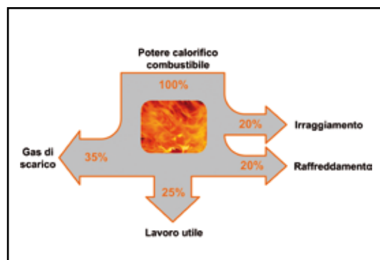
1.2 Rendimento motore a combustione interna
