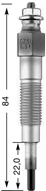
CZ 51 M 10 x 1.25 12 Hex 6,5 V
