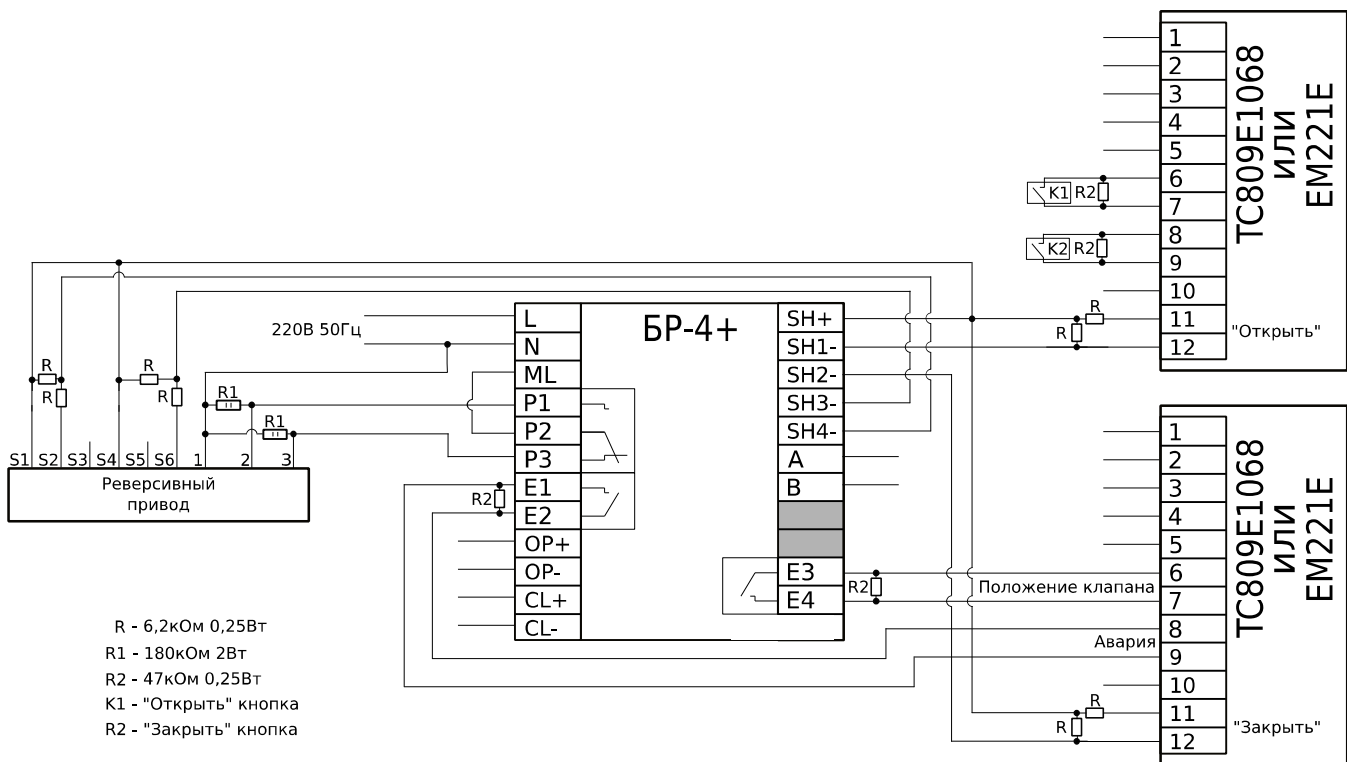
Рис. 5: Схема подключения «БР-4+» к адресным модулям адресно-аналоговой пожарной сигнализации для управления реверсивным приводом
