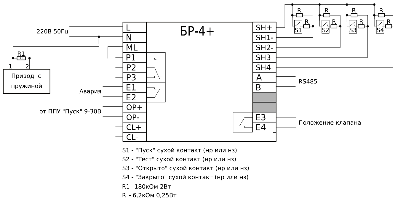
Рис. 3: Схема подключения привода с пружиной к «БР-4+» с контролем цепей управления и контроля
