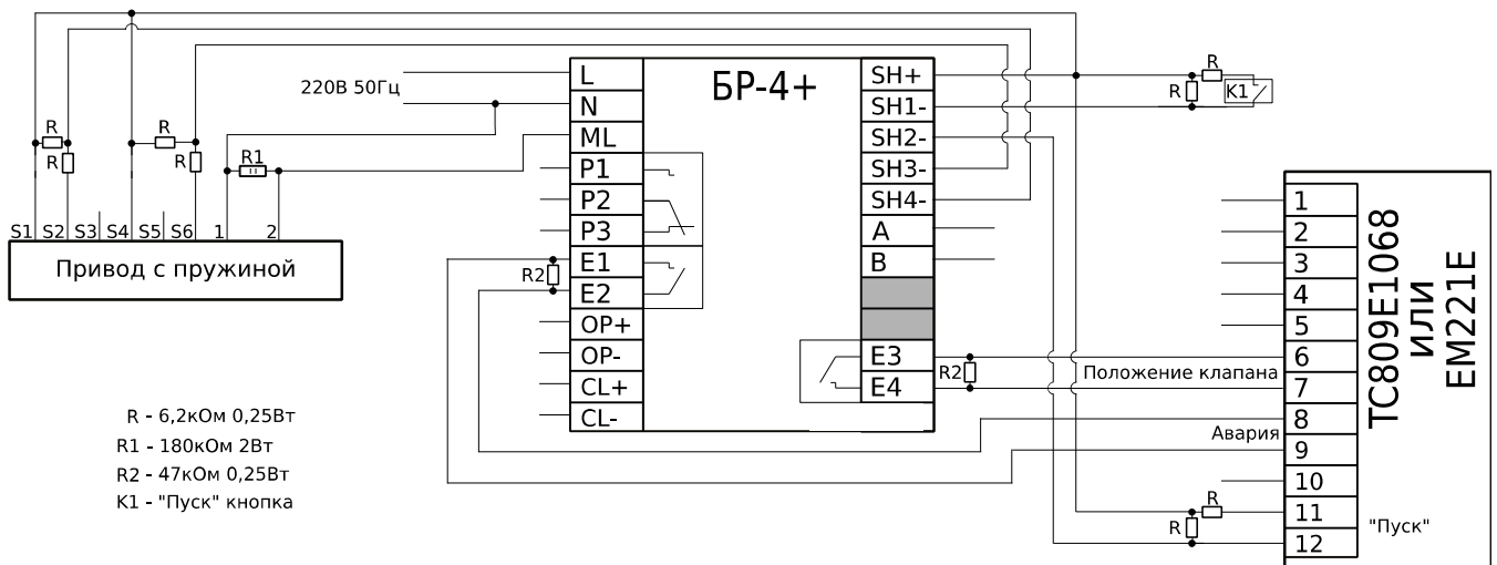
Рис. 6: Схема подключения «БР-4+» к адресному модулю адресно-аналоговой пожарной сигнализации для управления приводом с пружиной
