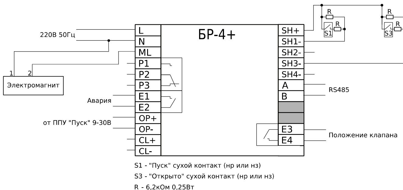
Рис. 4: Схема подключения электромагнитного привода к «БР-4+» с контролем цепей управления и контроля
