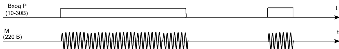
Д) Управление приводом дренажного клапана (повторитель сигнала на входе Р)
