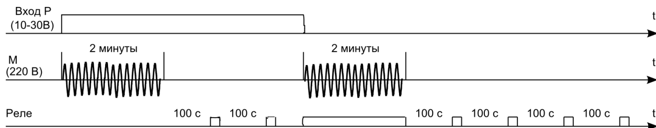
А) Управление реверсивным клапаном с контролем обеих обмоток привода каждые 100 сек переключением реле
