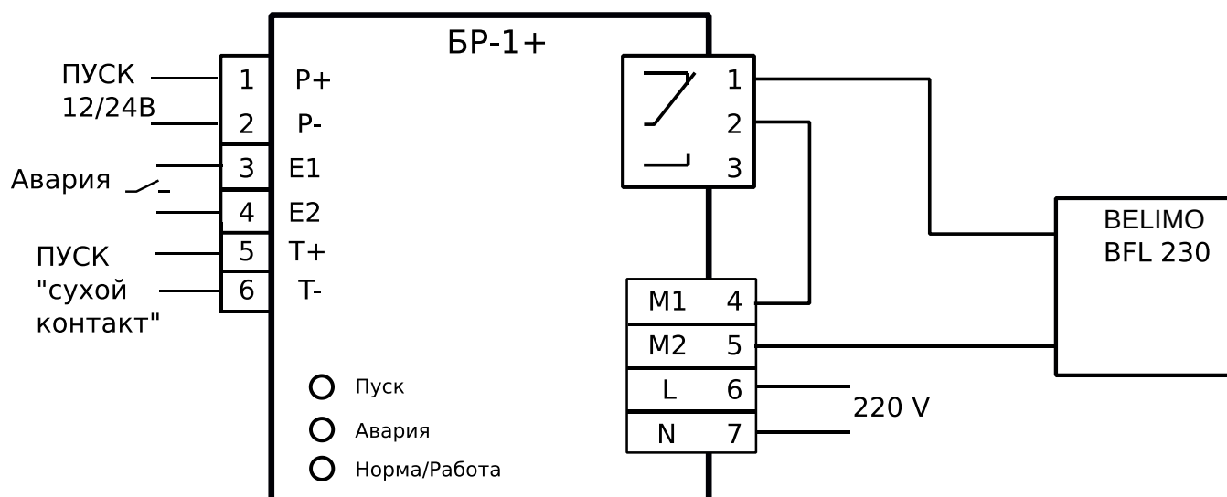
Рис. 10: Схема подключения привода типа BFL230 к блоку релейному «БР-1+»
