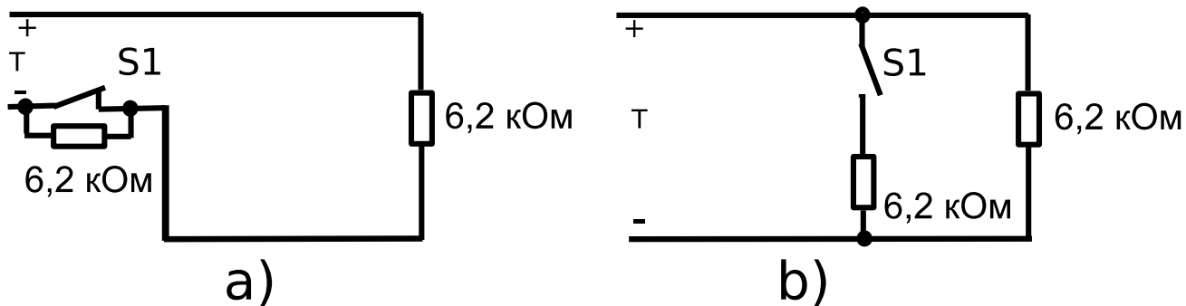
Рис. 4: Варианты включения механического переключателя S1 «Ручной пуск» в технологический шлейф «БР-1+».
