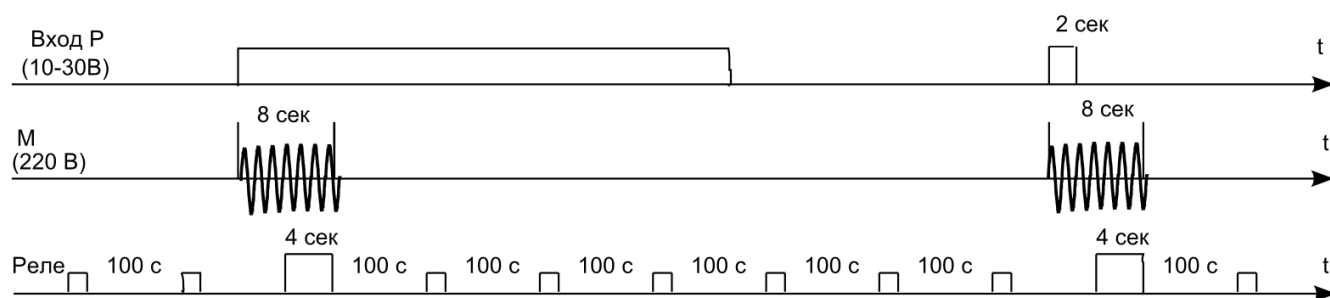
С) Управление двумя электромагнитными приводами
