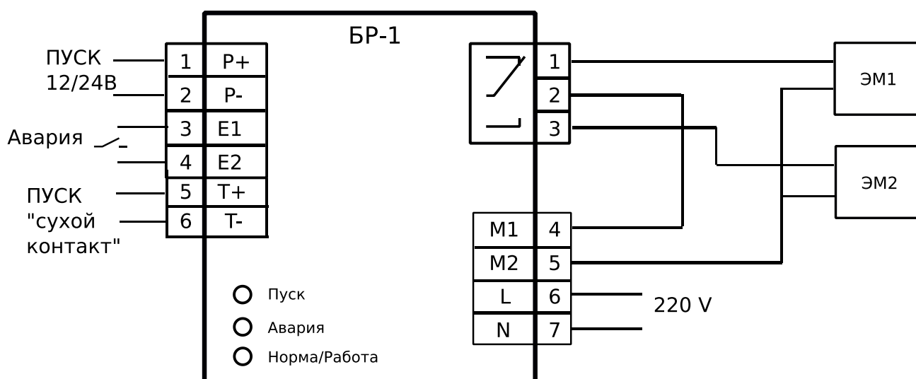
Рис. 6: Схема подключения двух электромагнитных приводов к «БР-1+».
