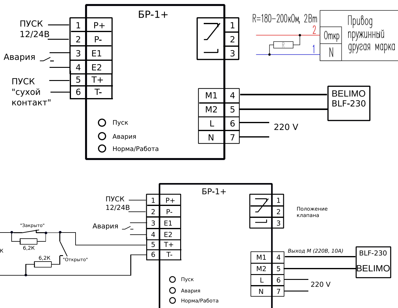
Рис. 7: Варианты подключения электромеханического привода с пружиной к «БР-1+».
