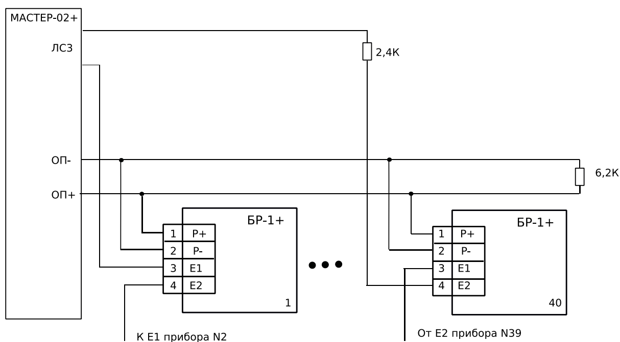
Рис. 8: Схема подключения «БР-1+» к прибору Мастер-02+.
