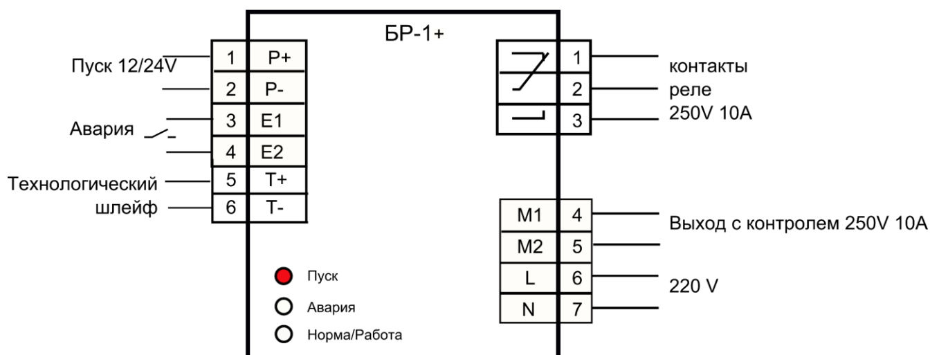
Рис. 1: Схема подключения «БР-1+»
