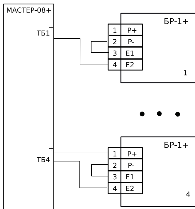
Рис. 9: Варианты схем подключения «БР-1+» к прибору Мастер-08+.
