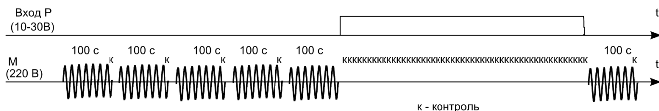
В) Управление приводом с пружиной
