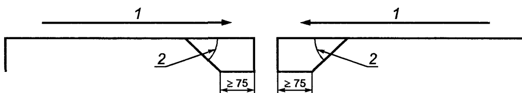
1 — направление закрывания створок дверей; 2 — угол \leq 45^\circ
