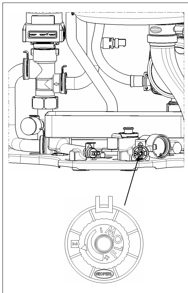
Ограничитель расхода
