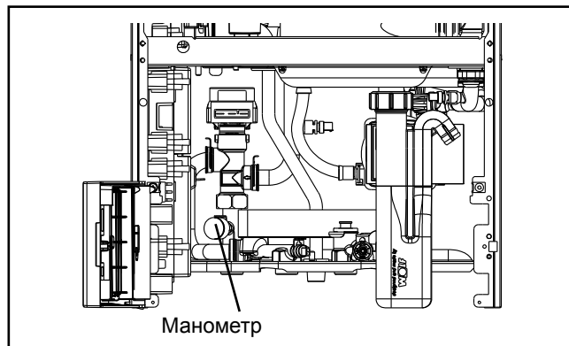
Манометр
